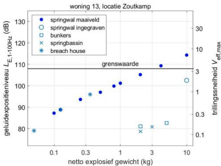
figuur 4-17 Illustratie van de resultaten van de berekeningen voor hinder door trillingen bij Kollumerwaard, voor een woning ten westen van het springterrein. De resultaten voor alle woningen staan in bijlage B.11
