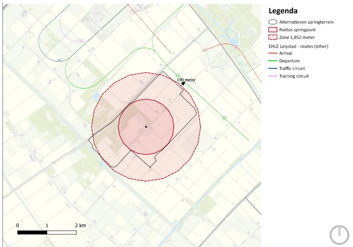
figuur 4-18 Springpunt met radius, de restrictieve 1 NM-zone (1.852 meter) voor het springterrein en de departure route voor Lelystad Airport
