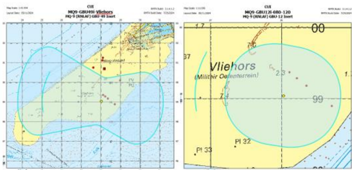
figuur 3-14: Benodigde veiligheidszone voor GBU-12 (links) en GBU-49 (rechts)
