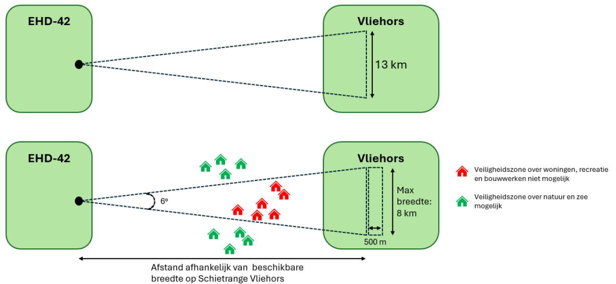
figuur 6-7: Principeweergave van de veiligheidszone die nodig is voor schietoefeningen richting Schietrange Vliehors. Boven de oorspronkelijke inschatting, onder de voor Zeef 2 bijgestelde inschatting.
