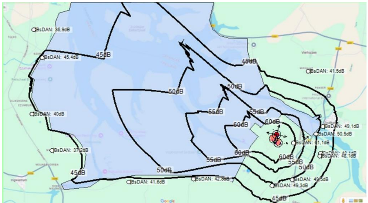
figuur 4-16 Berekende geluidniveaus Bs,dan bij de woningen voor de locatie bij Kollumerwaard, met de geluidcontouren (Bs,dan) van 45, 50, 55 en 60 dB.
