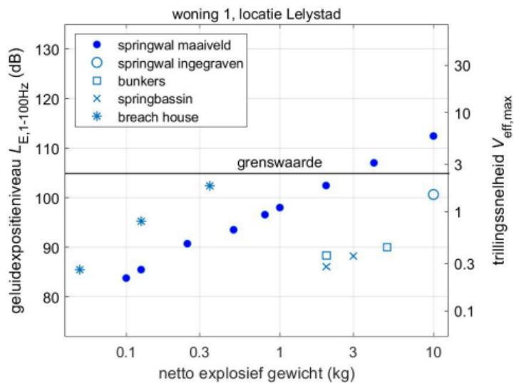
figuur 4-15 Illustratie van de resultaten van de berekeningen voor hinder door trillingen bij Lelystad voor een woning ten westen van het springterrein. De resultaten voor alle woningen staan in bijlage B.11
