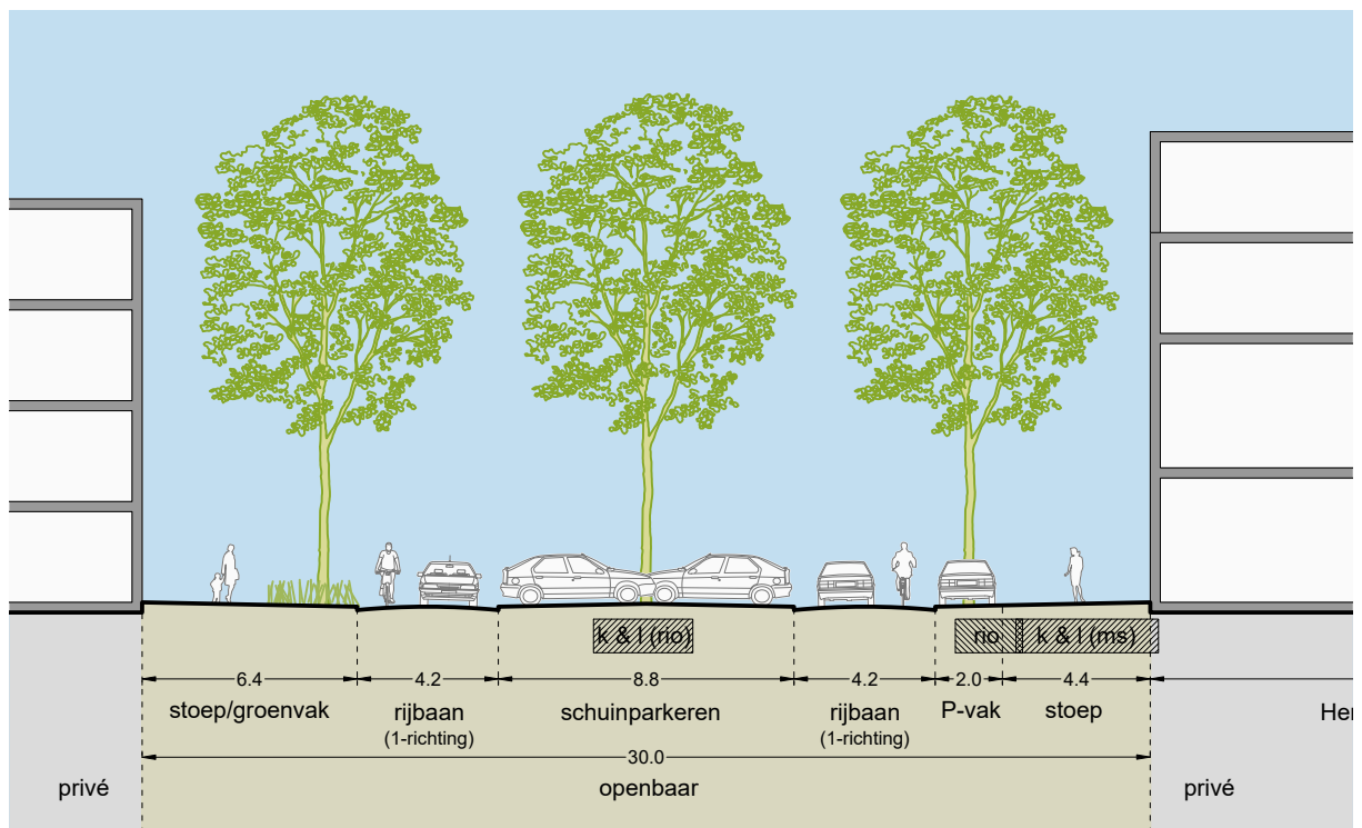
Doorsnede Herculesstraat
