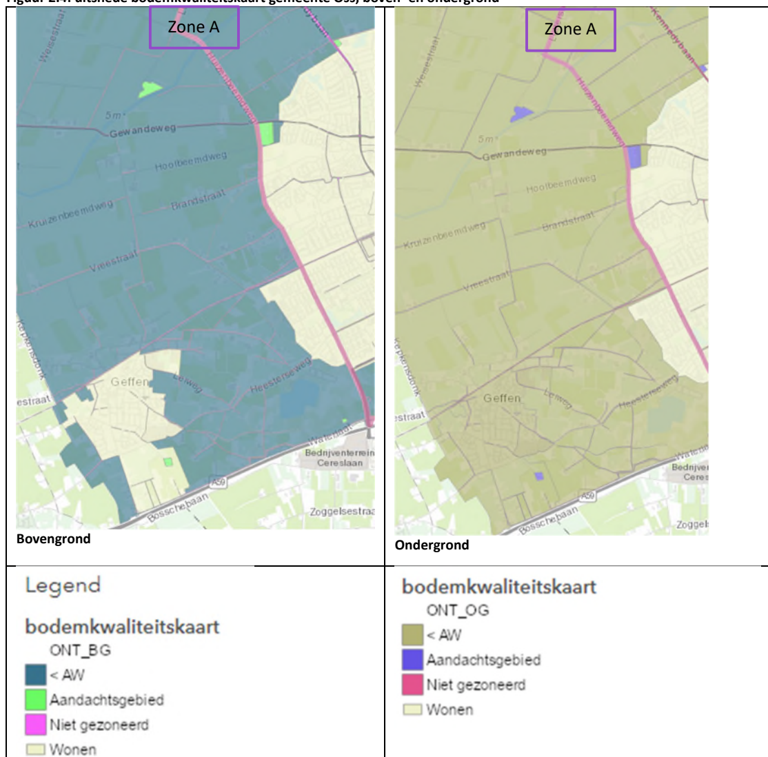
Figuur 2.4: uitsnede bodemkwaliteitskaart gemeente Oss, boven- en ondergrond
