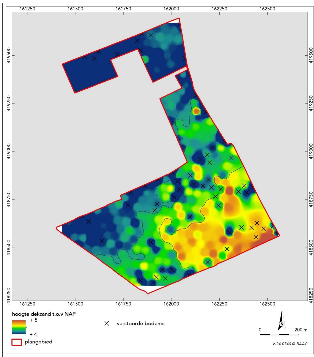
Afb. 3.4 Dekzanddieptekaart voor het plangebied met de hoogteligging van het dekzand. De oranjebruine tinten betreffen de hoogstgelegen delen, de donkerblauwe tinten de laaggelegen delen.
