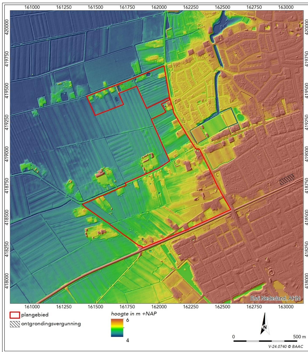
Afb. 2.3 Ligging van het plangebied en bekende ontgrondingslocaties (provincie Noord-Brabant 2024) op het Actueel Hoogtebestand (AHN4 2024).
