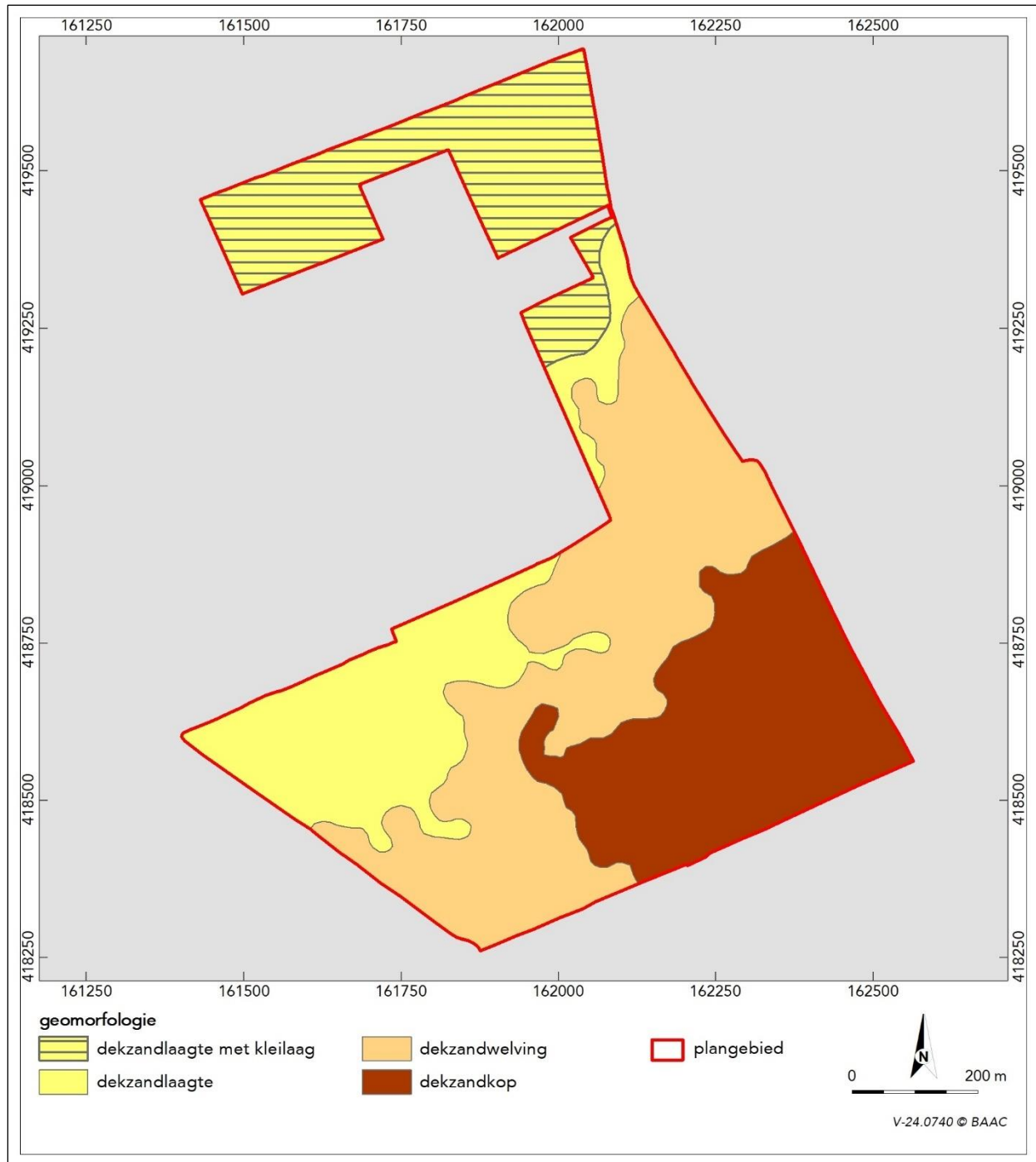
Afb. 3.5. Geomorfologische kaart van het plangebied.
