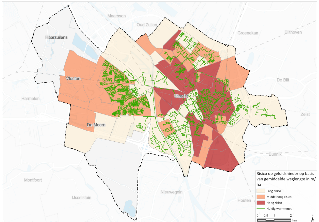
Figuur 5.7 Aantal meter weg per hectare, als indicator voor geluidshinder in de aanlegfase met bestaand warmtenet
