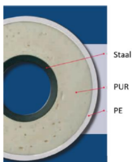
Figuur 5.18 Doorsnede van de veel gebruikte distributieleiding (VPS) voor een warmtenet
