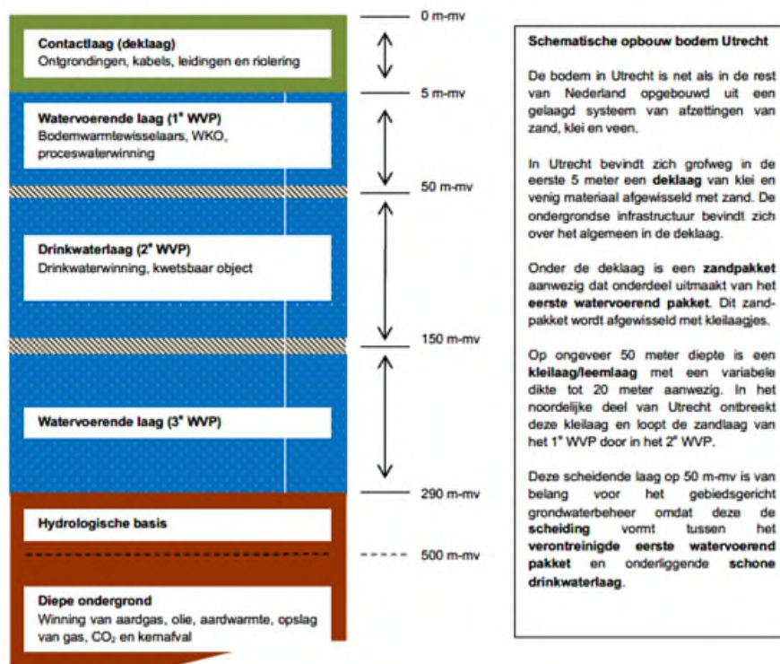
Figuur 5.17 Schematische weergave van de ondergrond van de gemeente Utrecht (Bron: Gebiedsplan ggb, 2015)
