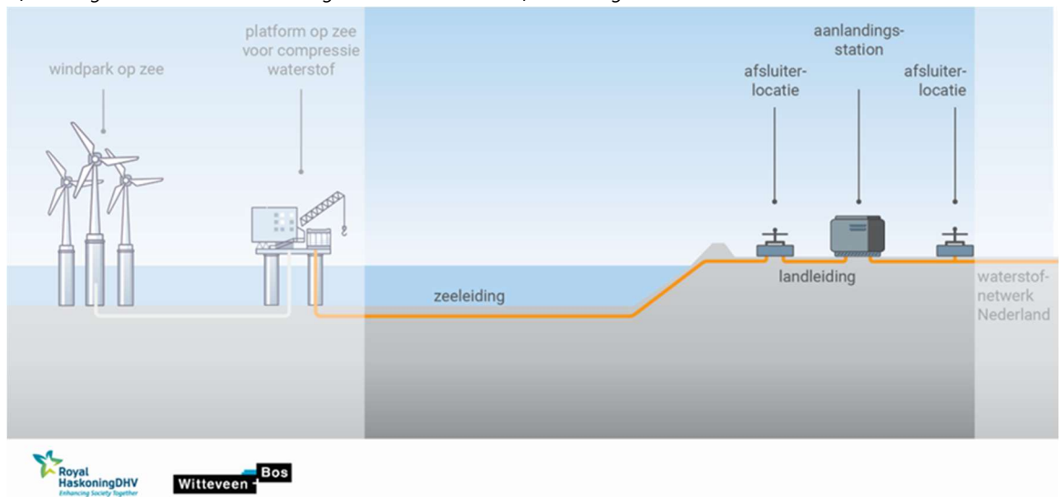
Afbeelding 1.4 - Schematische weergave van een waterstofverbinding
