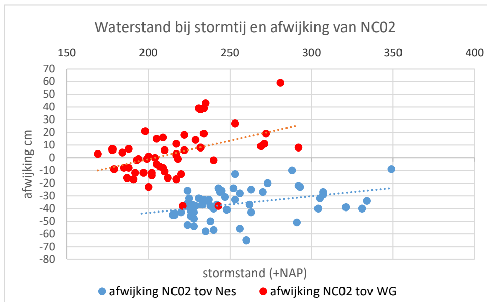
Figuur 14. Afwijking van de hoogste waterstand in vallei NC02 ten opzichte van de RWS meetpalen Nes en Wierumergronden.
