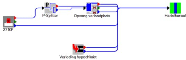
Figuur 4.3: Lozingspad hypochloriet naar Hartelkanaal
