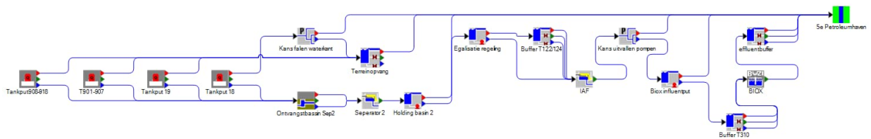
Figuur 4.4: Lozingspad separator 2 via IAF/BIOX.
