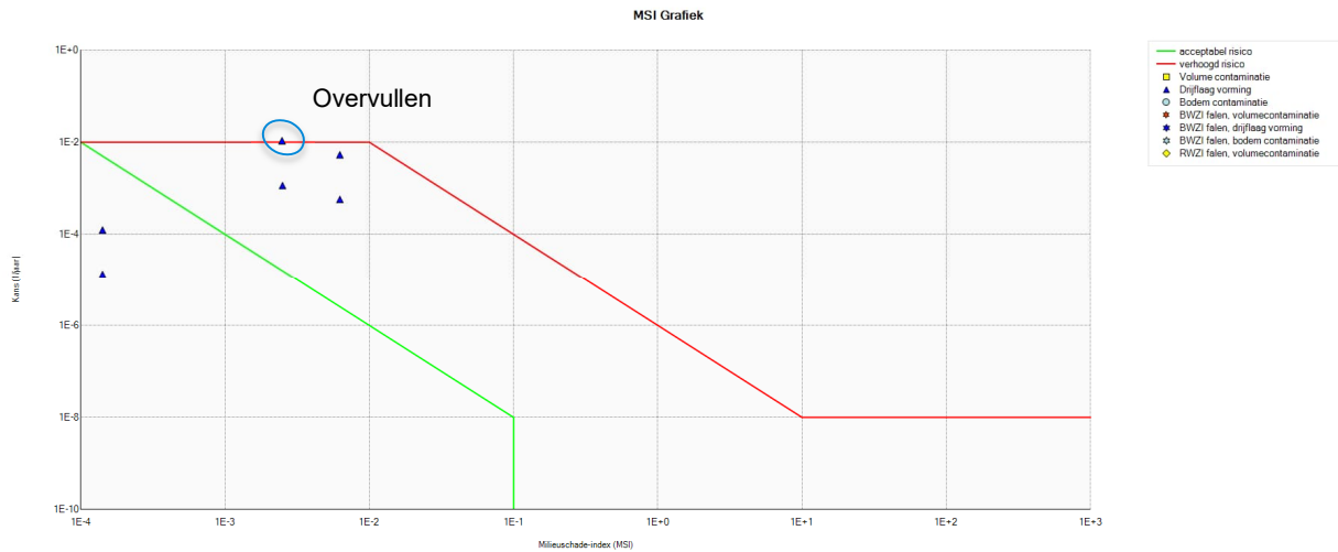
Figuur 5.5: MSI grafiek binnenvaart jetty 4.
