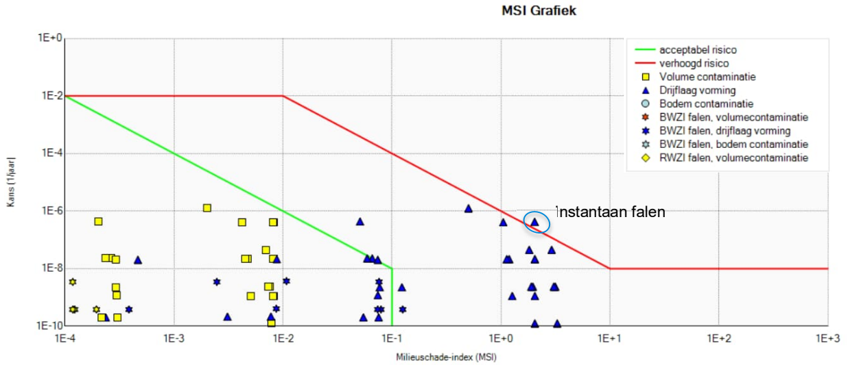
Figuur 5.11: MSI grafiek bulkopslag (tankput 6)
