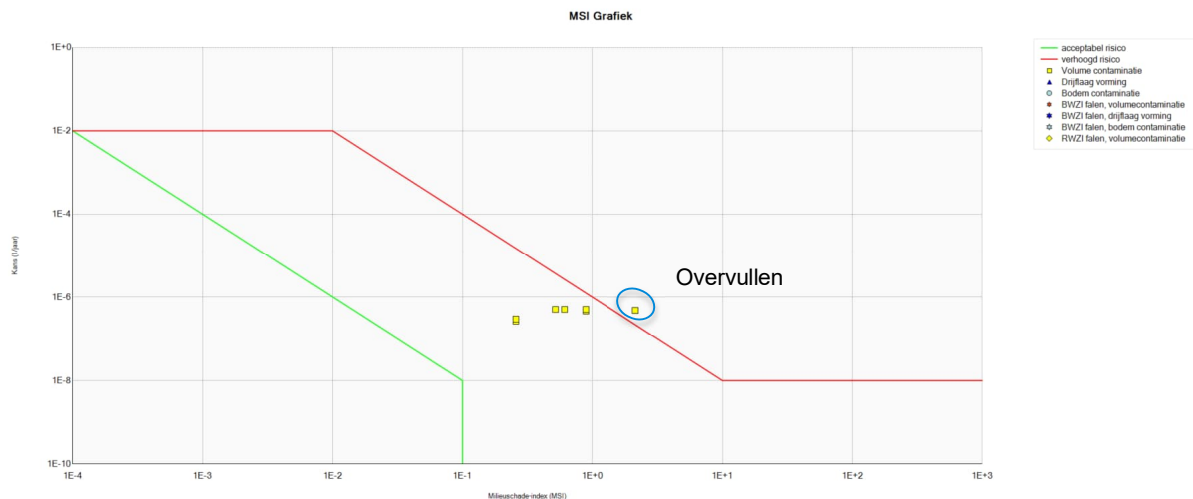
Figuur 5.7: MSI grafiek 2170F (hypochloriet tank met handbediende afsluiter naar Hartelkanaal).
