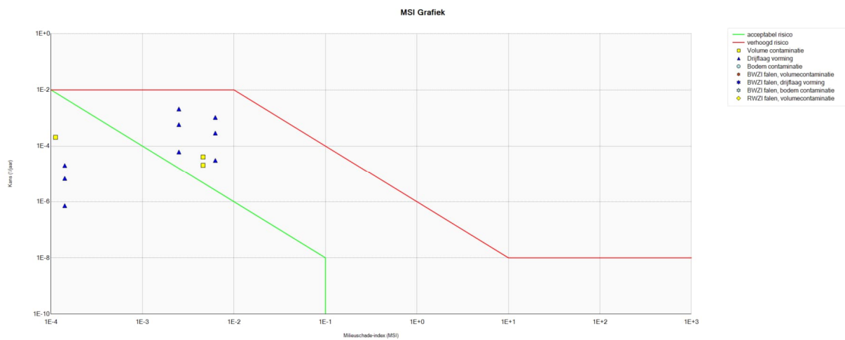
Figuur 5.6: MSI grafiek binnenvaart jetty 2.
