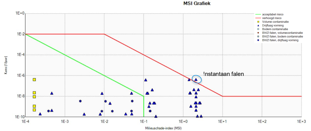
Figuur 5.12: MSI grafiek bulkopslag (tankput 7)
