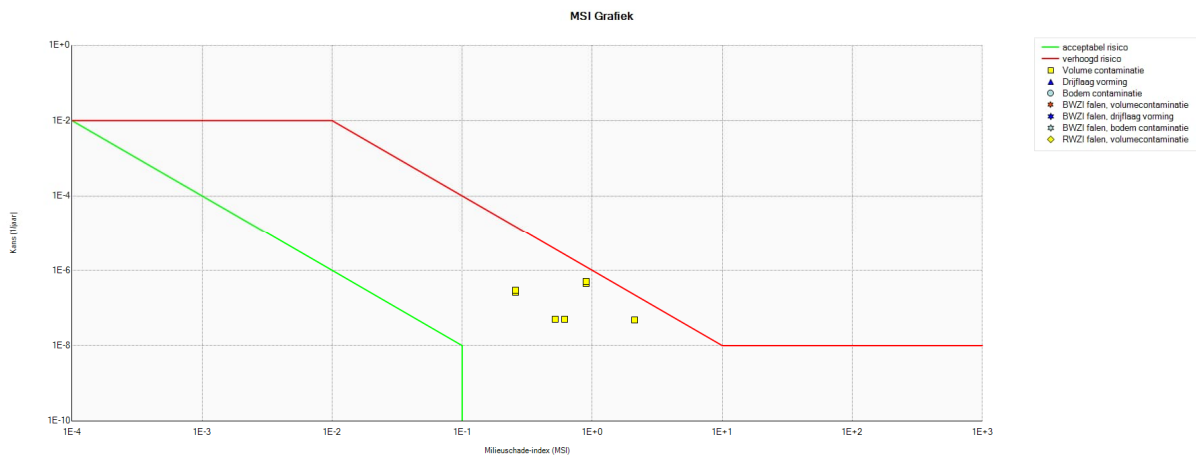
Figuur 5.8: MSI grafiek 2170F (hypochloriet tank met automatisch gestuurde afsluiter naar Hartelkanaal).
