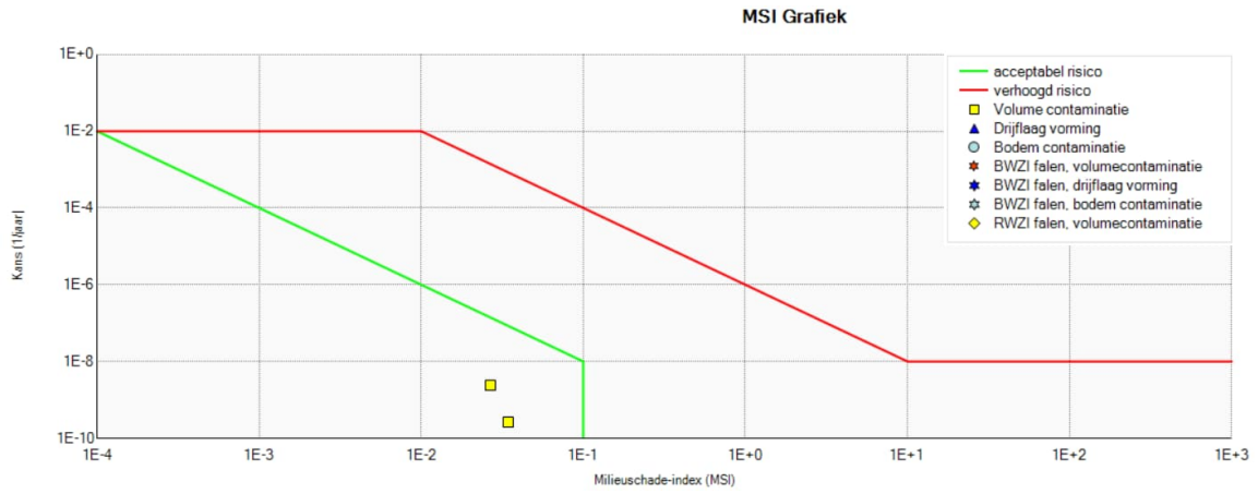
Figuur 5.23: Risico's tankwagenverlading citroenzuur.
