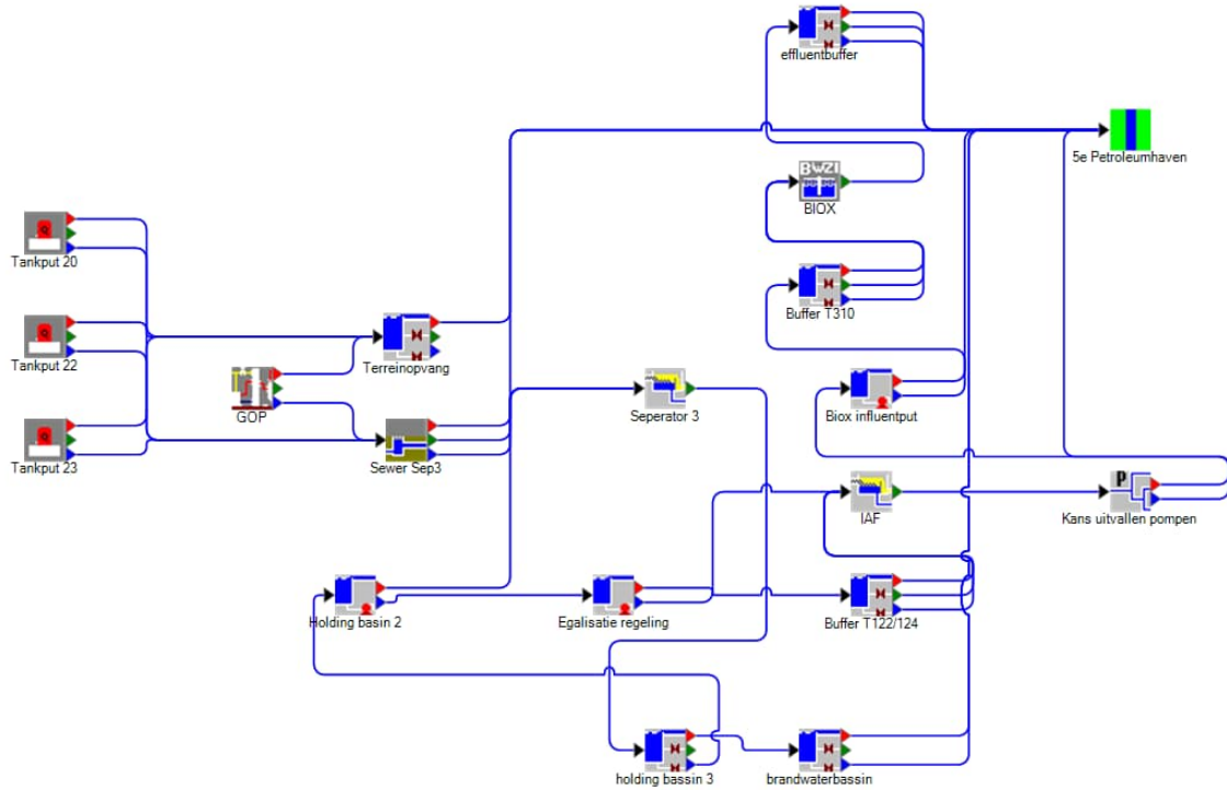
Figuur 4.1: Lozingspad separator 3
