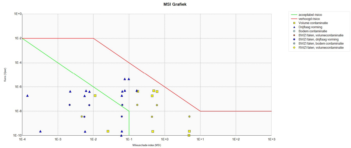
Figuur 5.19. Tank 905 (treated feedstock 4000m 3 ). Identiek aan T-906.
