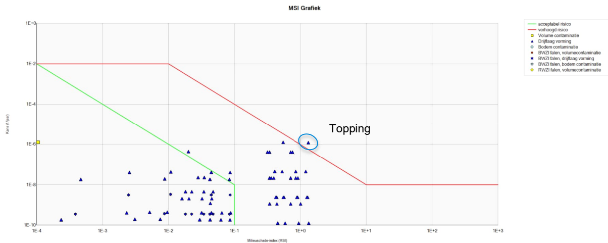
Figuur 5.13: MSI grafiek bulkopslag (tankput 10)
