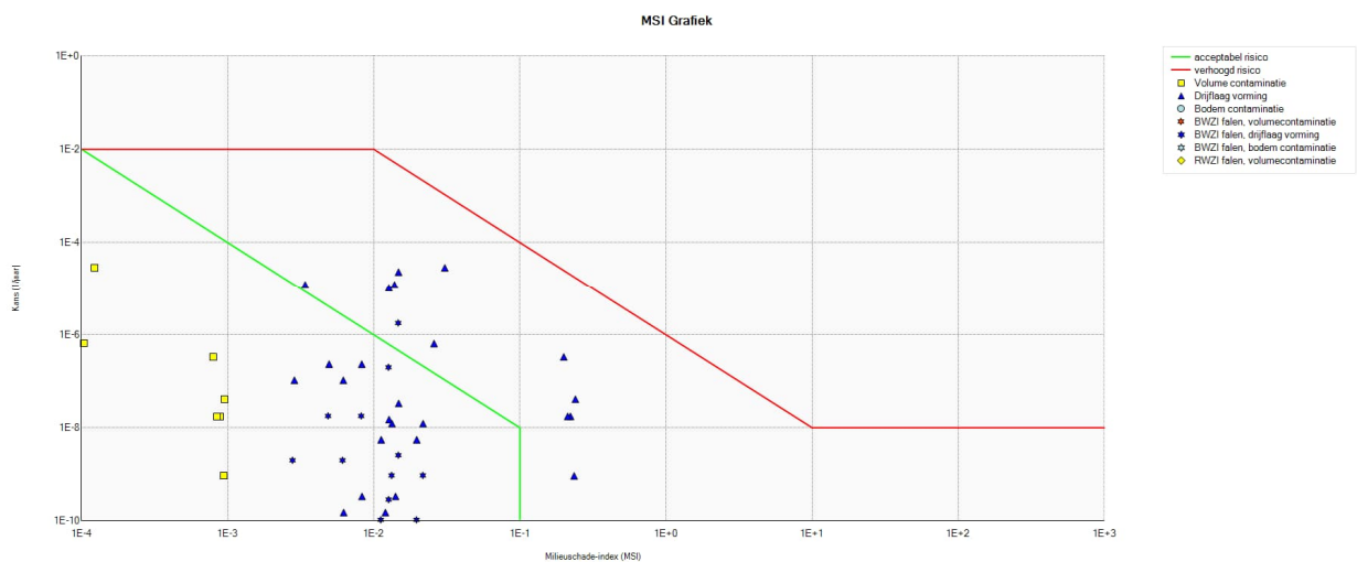
Figuur 5.4: MSI grafiek leidingen
