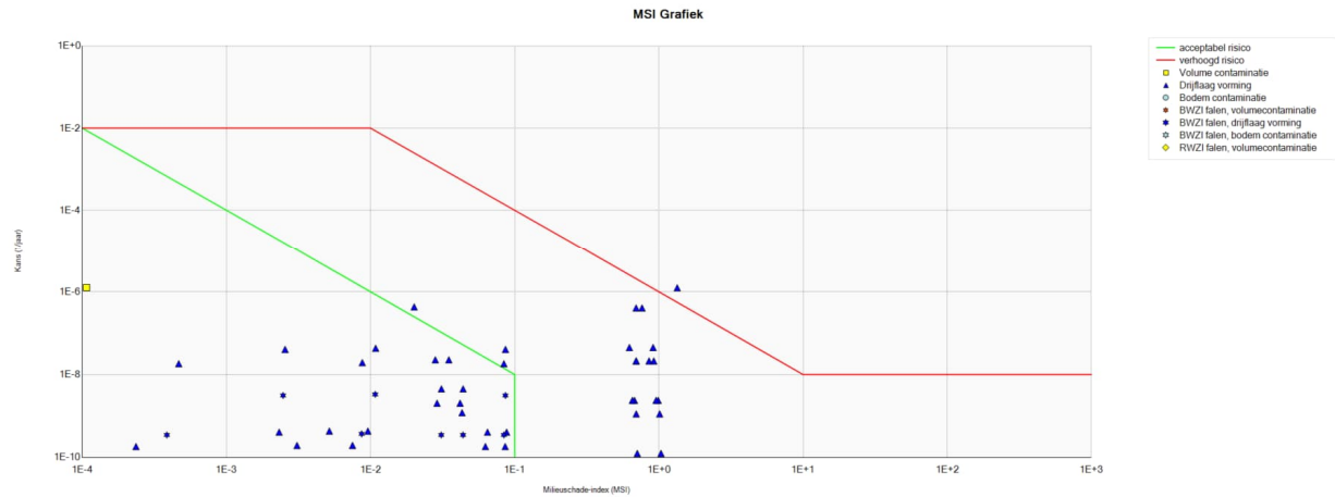
Figuur 5.21. Tank 915 in tankput 10. Identiek aan T-916 (Topping scenario, zie Figuur 5.13).
