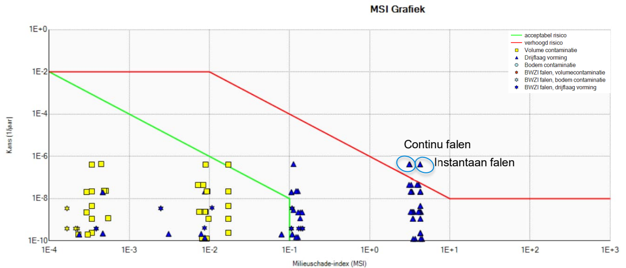
Figuur 5.15: MSI grafiek bulkopslag (tankput 1)
