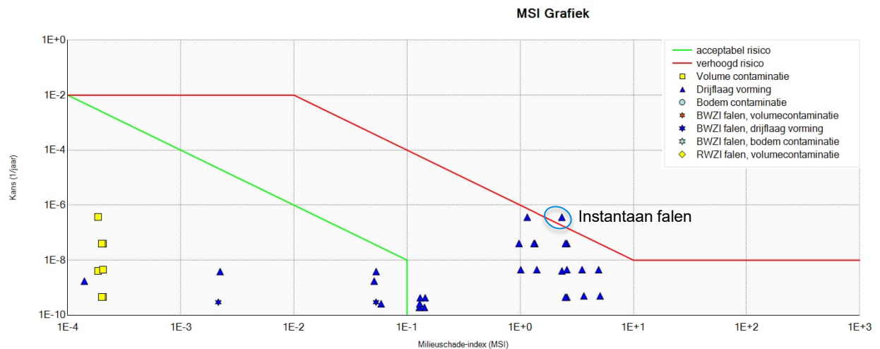
Figuur 5.16: MSI grafiek bulkopslag (tankput 25)
