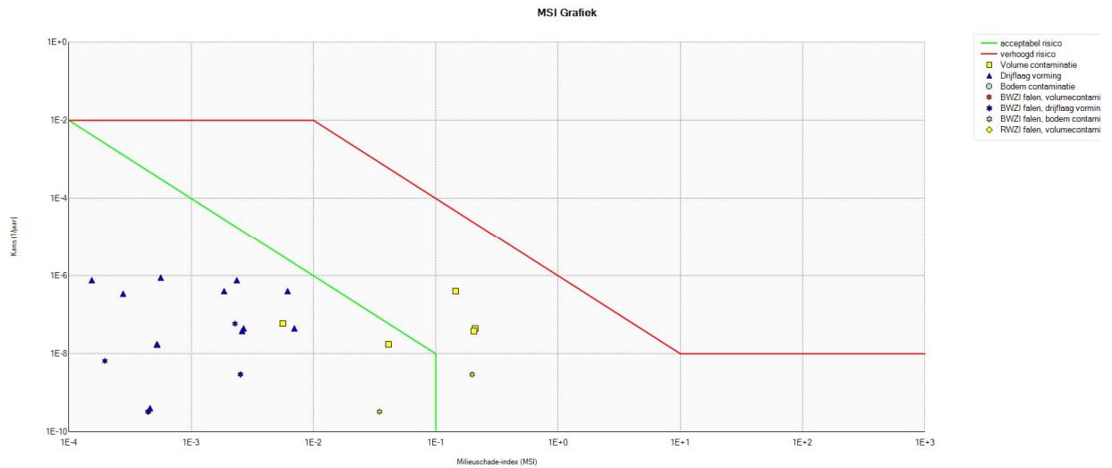
Figuur 5.3: MSI grafiek productie units GOP
