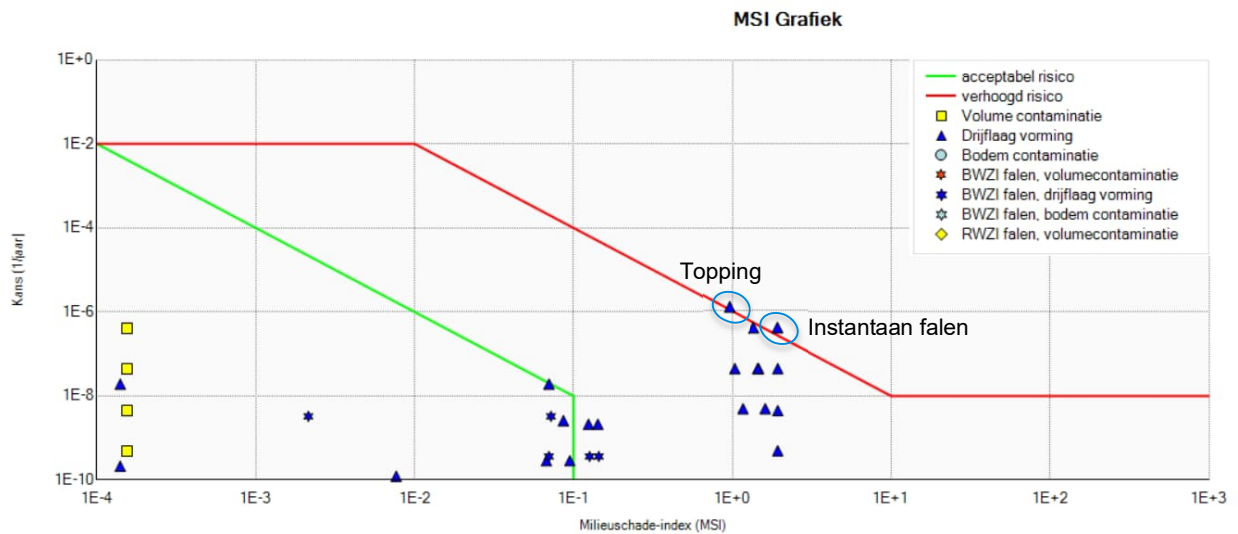
Figuur 5.9: MSI grafiek bulkopslag (tankput 18, tank 333)
