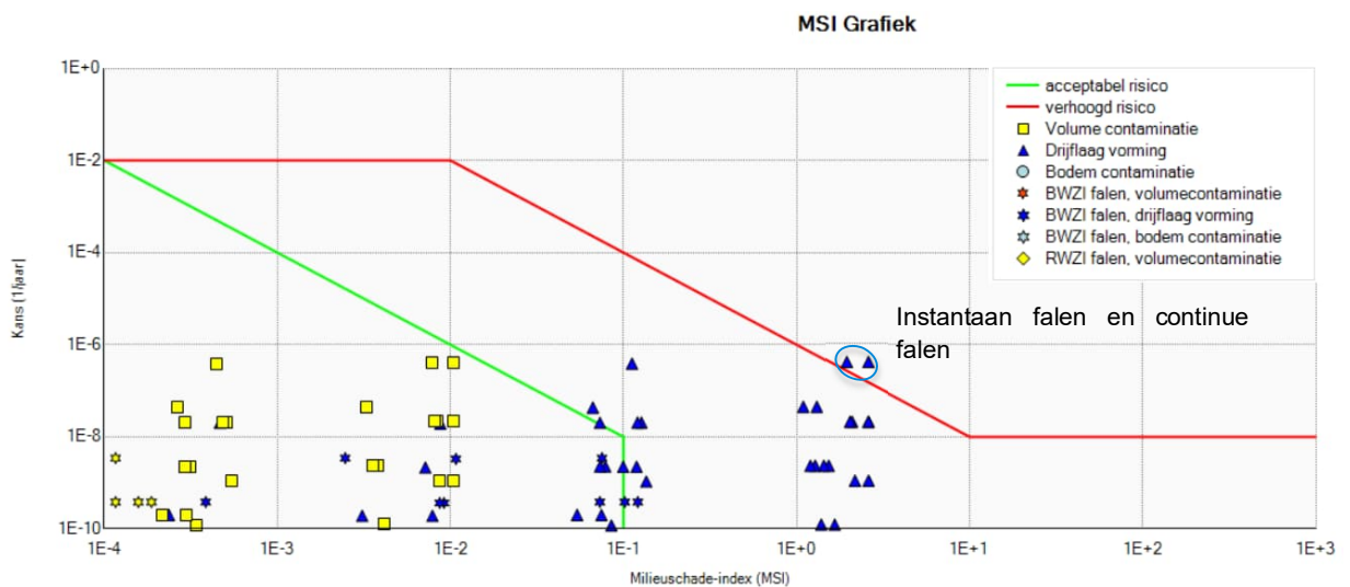
Figuur 5.10: MSI grafiek bulkopslag (tankput 5)
