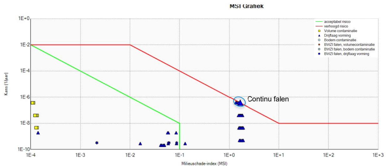
Figuur 5.14: MSI grafiek bulkopslag (tankput 23)
