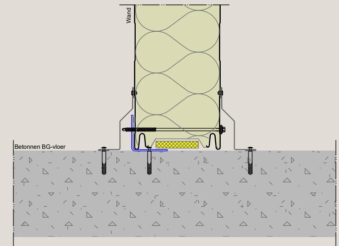
Principedetail scheidingswand
