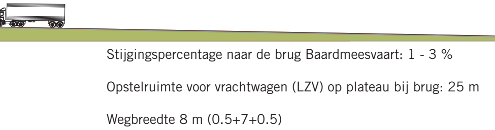
PROFIEL G-G'
