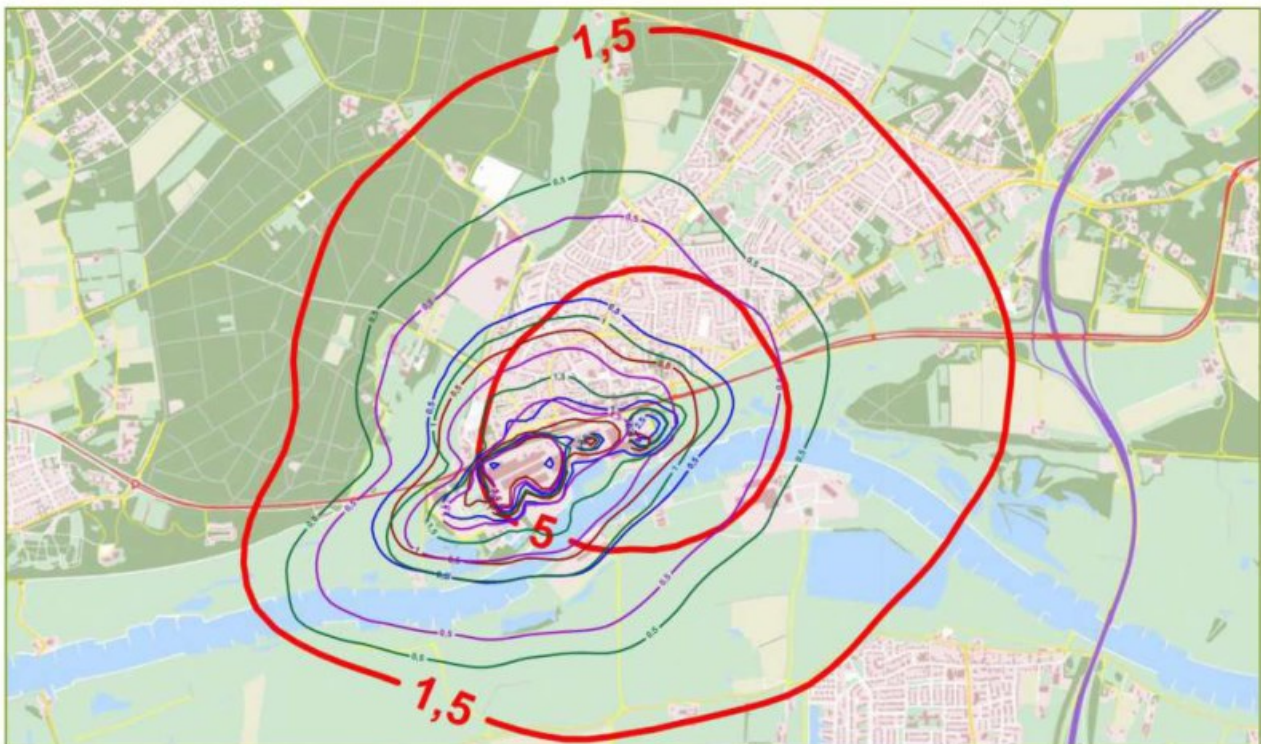
Figuur 4.5: Geurbelasting SK Parenco als geurcontouren in ouE/m^3 als 98-percentiel – Alternatieven t.o.v. de referentiesituatie
