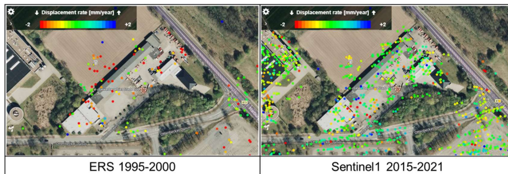
Figuur 7: Weergave van de bodemdalingssnelheid op basis van INSAR-data gedurende 1995-2000 en 2015-2021 boven caveerne Stade T5 (bron: SkyGeo portal voor Nobian). Dit gebied is gekozen omdat het het centrum van het bodemdalingsgebied was, caveerne T5 ook de grootste caveerne was, en de gebouwen sinds 1995 onveranderd zijn, waardoor de data uit beide periodes goed vergelijkbaar is. Te zien is dat in de periode 1995-2000 bodemdaling plaatsvond met een snelheid van 2 mm/jaar. Destijds was het winningsgebied nog in bedrijf. Waterpasgegevens geven een vergelijkbaar beeld. In de periode 2015-2020 (10-15 jaar na abandonment van de putten) is de bodemdalingssnelheid 0 mm/jaar.
