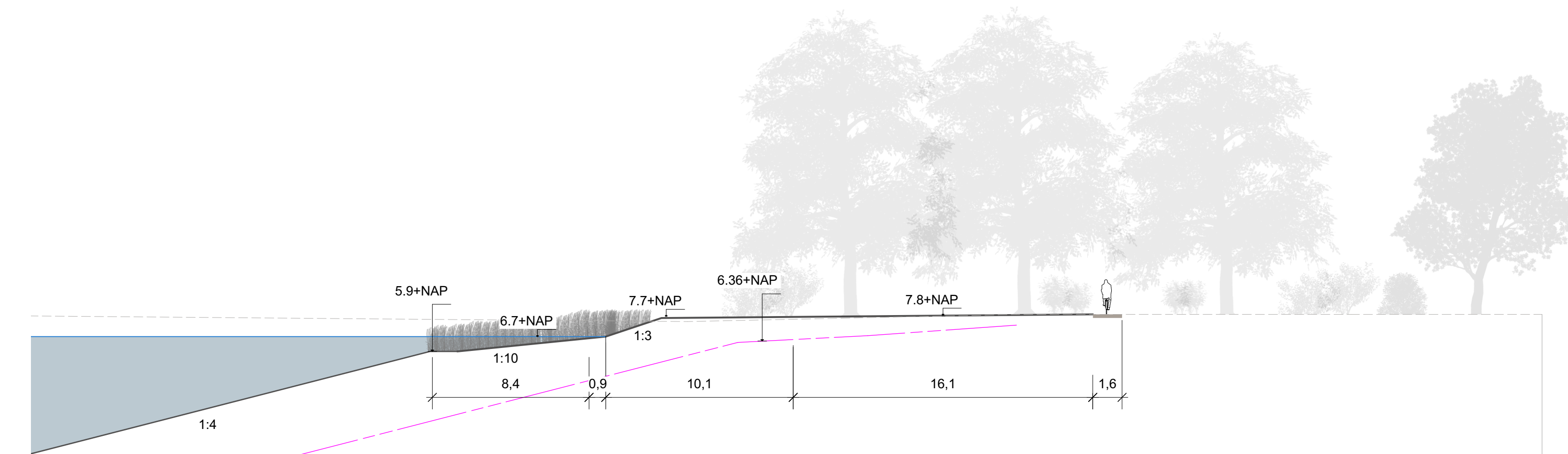
Oostrand - noord Scale: 1:200
