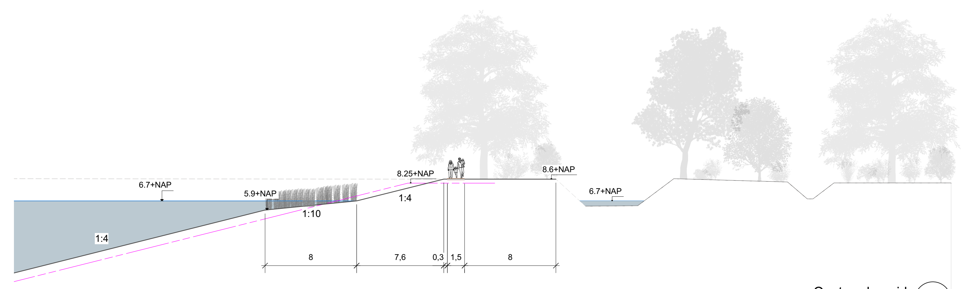
Oostrand - zuid Scale: 1:200
