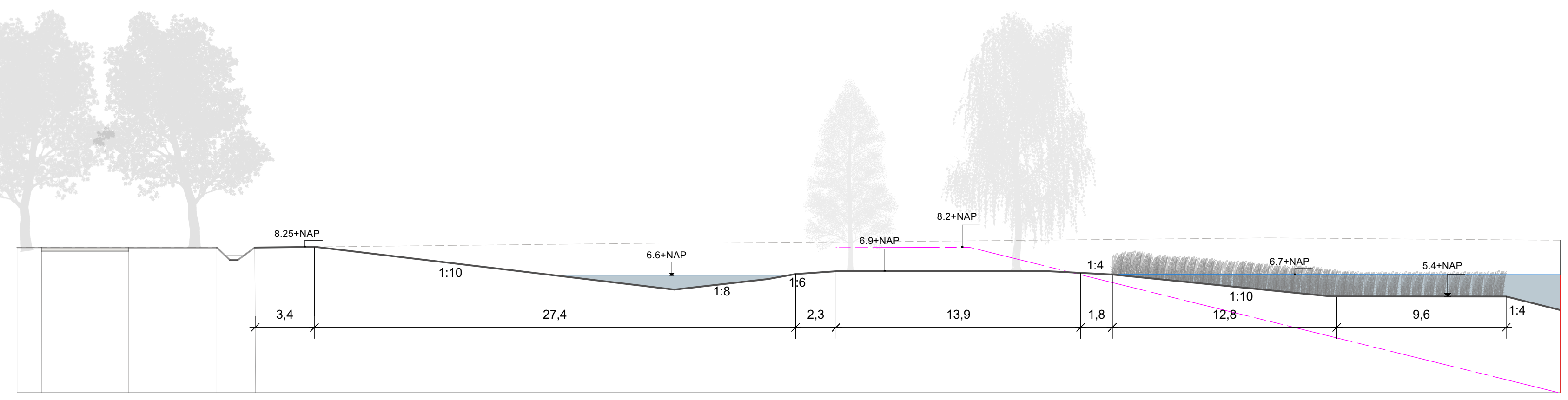
1 Westrand - Noord Scale: 1:200
