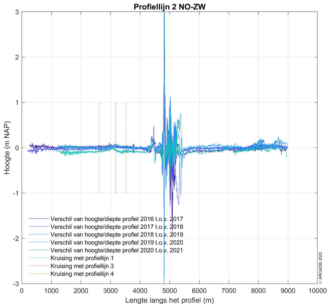
Figuur 5-6 Verschilplot langs profiellijn 2 van noordoost naar zuidwest voor de hoogte/diepte raai meetgegevens tussen 2016 t.o.v. 2017, 2017 t.o.v. 2018, 2018 t.o.v. mei 2019, 2019 t.o.v. 2020 en 2020 t.o.v. 2021. Een positieve waarde betekent dat de hoogte/diepteraai van het opvolgende jaar hoger ligt dan de hoogte/diepteraai van het eerdere jaar.
