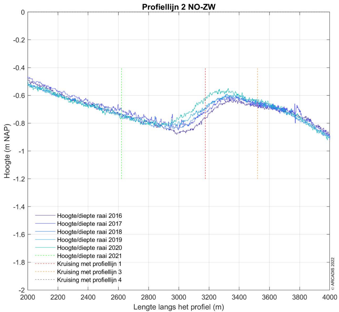
Figuur 5-5 Ingezoomd dwarsprofiel langs profiellijn 2 van noordoost naar zuidwest voor de hoogte/diepte raai meetgegevens van 2016, 2017, 2018, 2019, 2020 en 2021 (Detail van Figuur 5-4).
