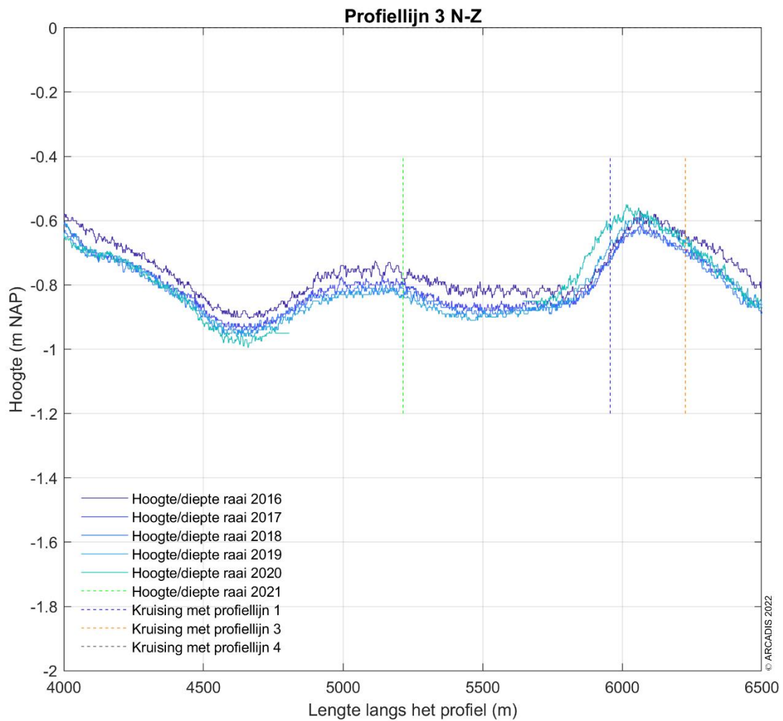
Figuur 5-8 Ingezoomd dwarsprofiel van de Ballastplaat langs profiellijn 3 van noord naar zuid voor de hoogte/diepte raai meetgegevens van 2016, 2017, 2018, 2019, 2020 en 2021 (Detail van Figuur 5-7).
