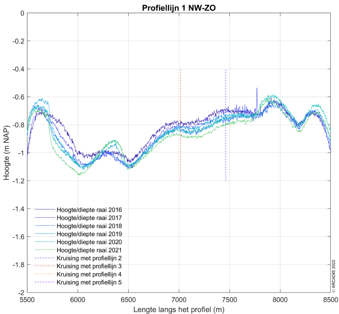
Figuur 5-2 Ingezoomd dwarsprofiel van de Ballastplaat langs profiellijn 2 van noordwest naar zuidoost voor de hoogte/diepte raai meetgegevens van 2016, 2017, 2018, 2019, 2020 en 2021 (Detail van Figuur 5-1).
