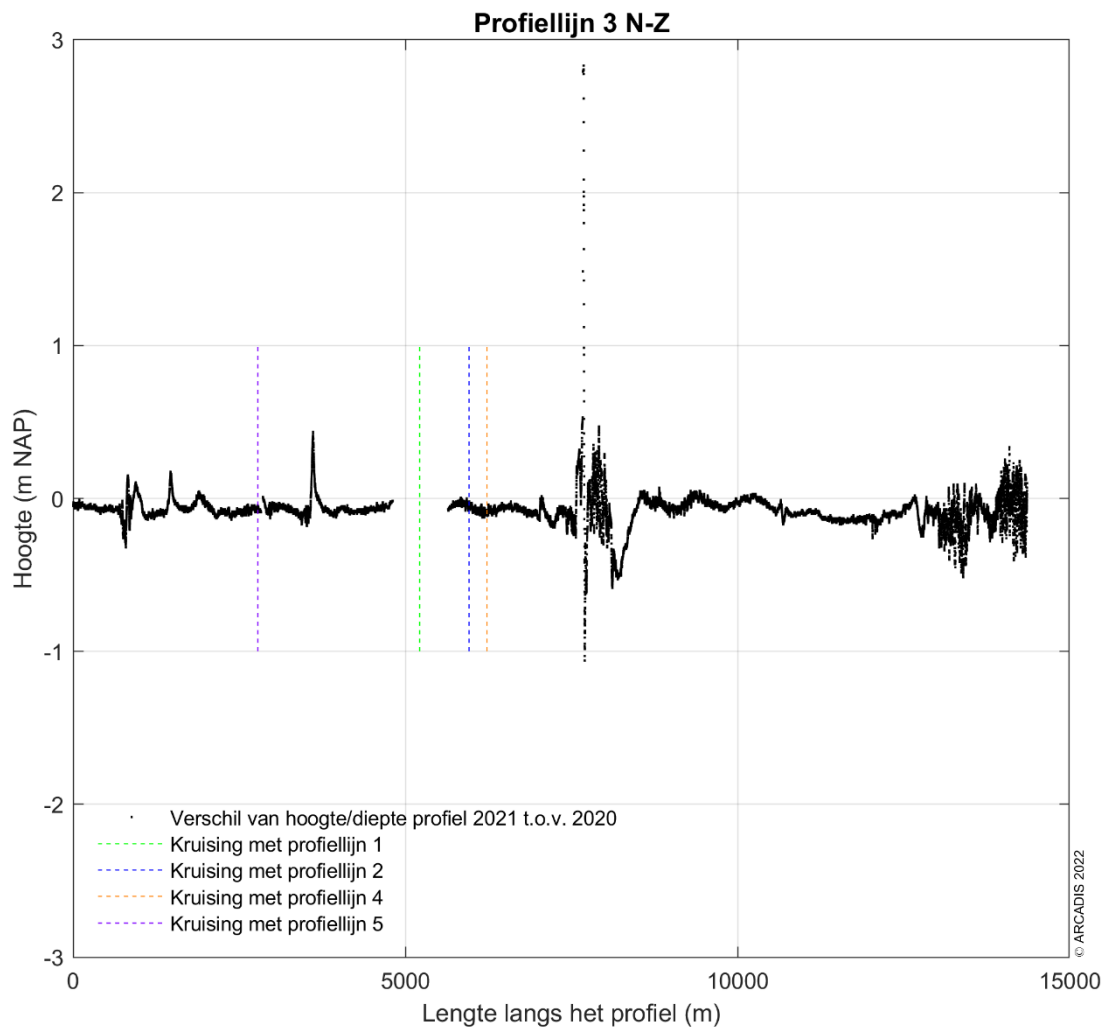
Figuur 4-53 Verschilplot langs profiellijn 3 van noord naar zuid voor de hoogte/diepte raai meetgegevens van 2020 en 2021. Een positieve waarde betekent dat de hoogte/diepteraai van mei 2021 hoger ligt dan de hoogte/diepteraai van 2020.
