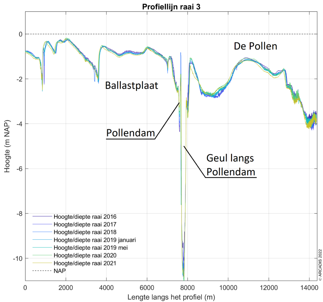
Figuur 5-7 Dwarsprofiel langs profiellijn 3 van noord naar zuid voor de hoogte/diepte raai meetgegevens van 2016, 2017, 2018, 2019, 2020 en 2021.
