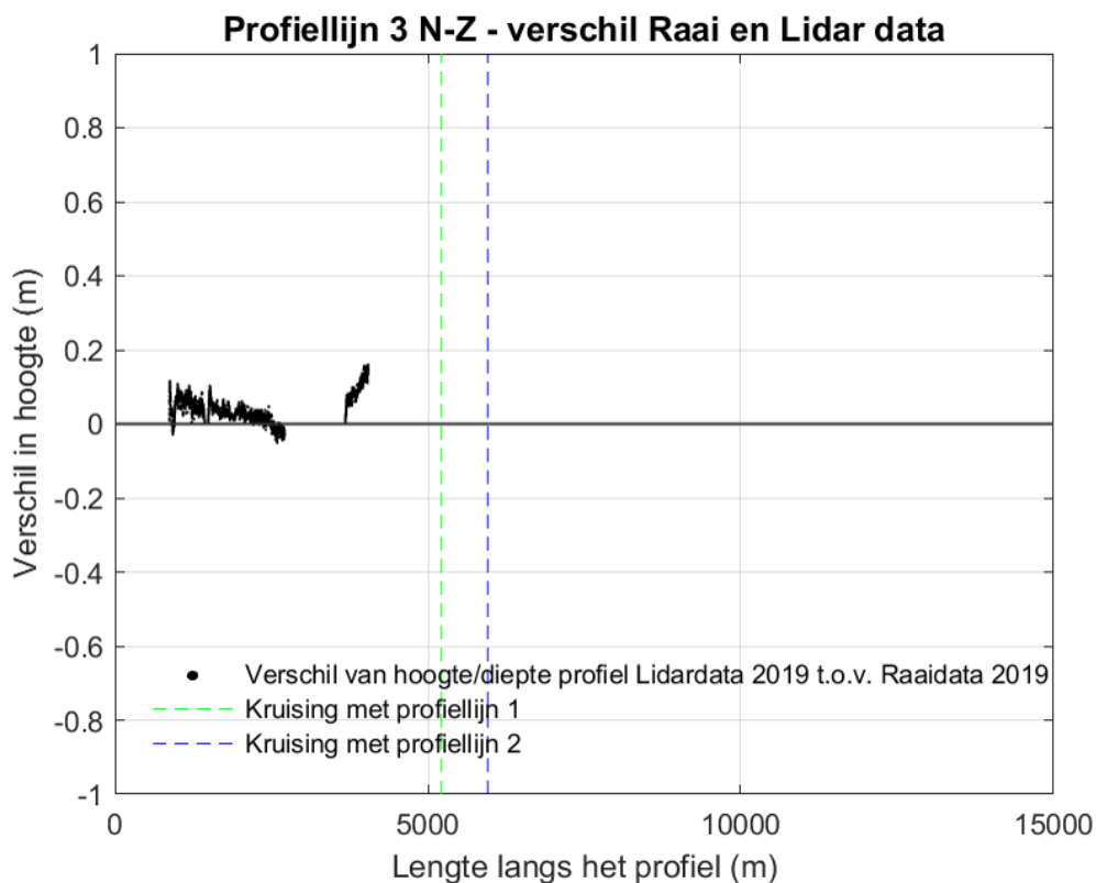
Figuur 0-22 Verskilplot langs profiellijn 3 van noord naar zuid voor de hoogte/diepte raai meetgegevens van 2019 en de LiDAR-data van 2019. Een positieve waarde betekent dat de LiDAR lager ligt dan de hoogte/diepteraai.
