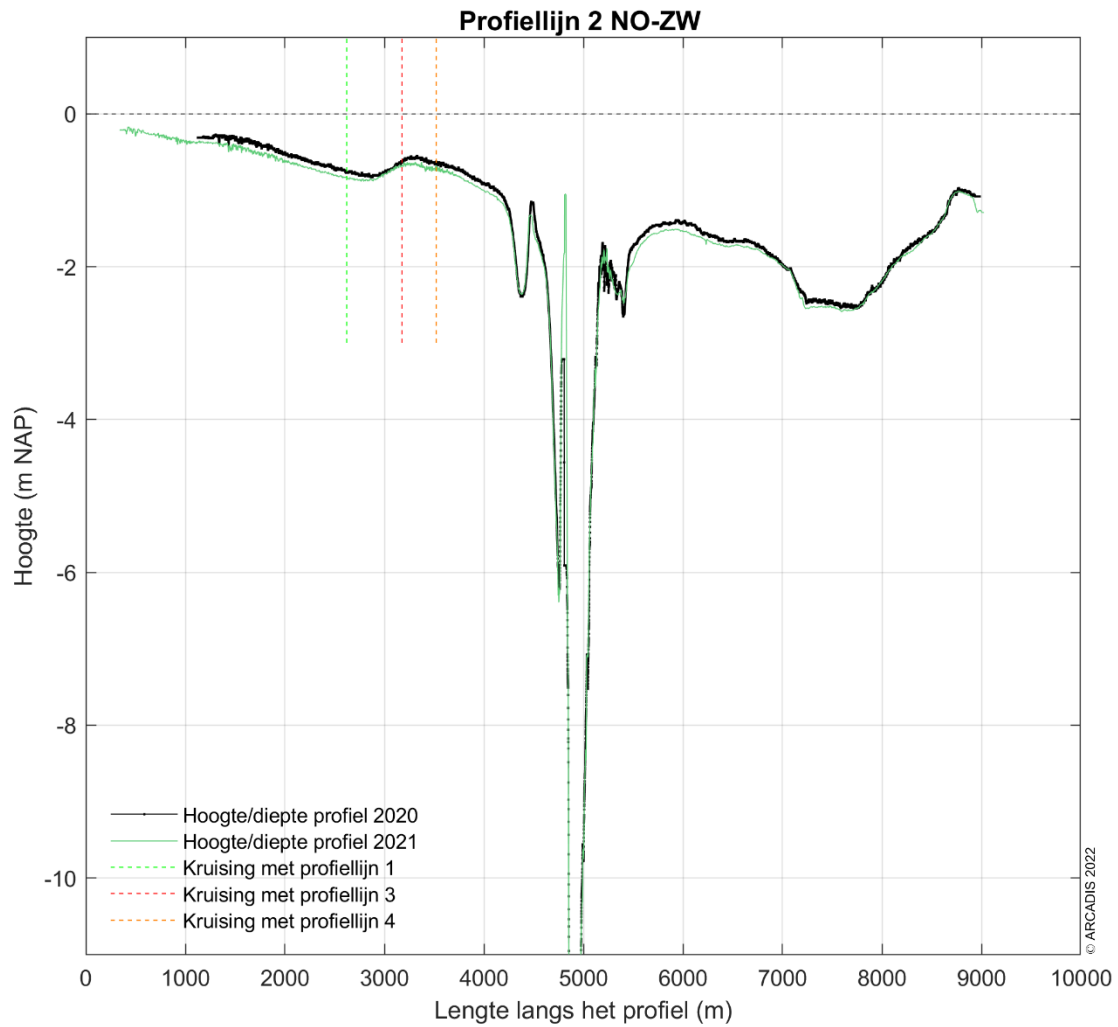
Figuur 4-49 Dwarsdoorsnede langs profiellijn 2 van noordoost naar zuidwest voor de hoogte/diepte raai meetgegevens van 2020 en 2021.
