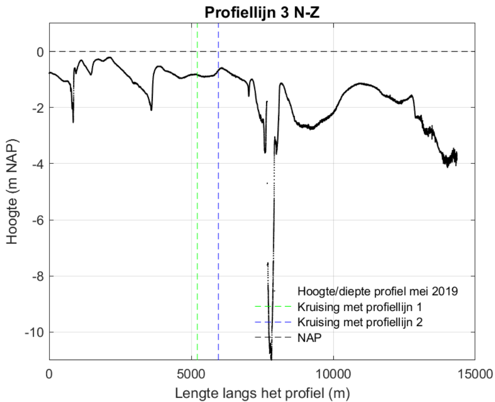
Figuur 3-29 Dwarsdoorsnede langs profielijn 3 van noord naar zuid in mei 2019.
