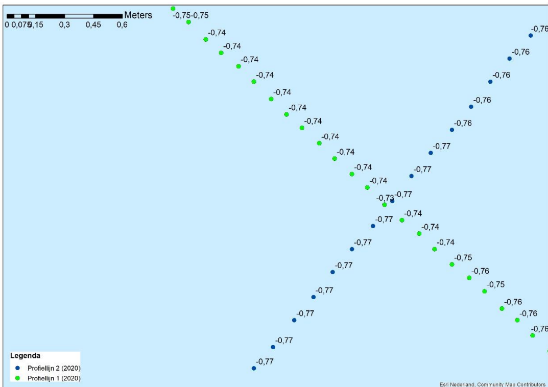
Figuur 3-30 Detailkaart controlepunt tussen profielijn 1 en profielijn 2 voor de hoogte/diepte raaien mei 2019, hoogtemetingen zijn weergegeven in m NAP.
