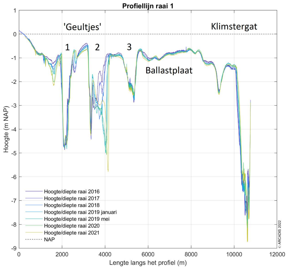
Figuur 5-1 Dwarsprofiel langs profiellijn 1 van noordwest naar zuidoost voor de hoogte/diepte raai meetgegevens van 2016, 2017, 2018, 2019, 2020 en 2021.
