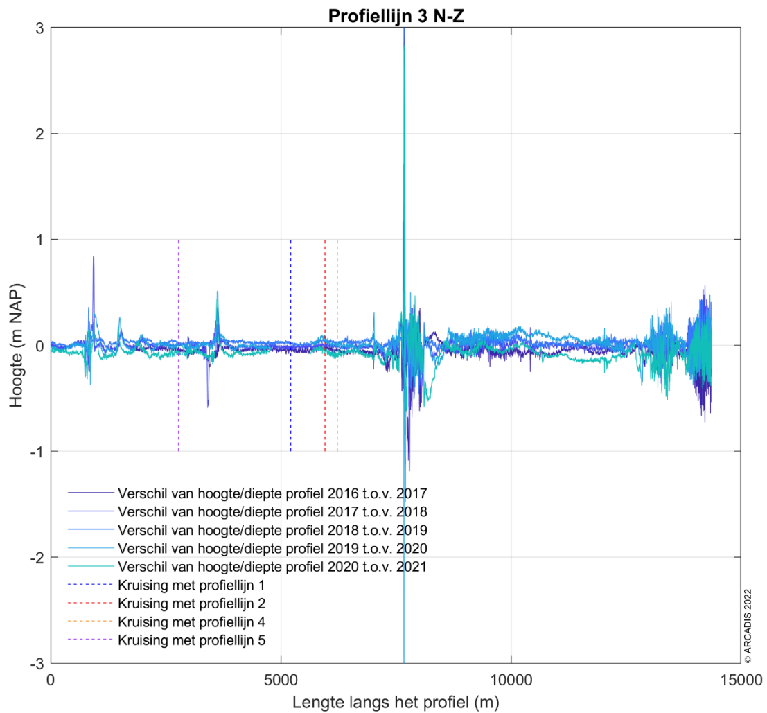
Figuur 5-9 Verschilplot langs profiellijn 3 van noord naar zuid voor de hoogte/diepte raai meetgegevens tussen 2016 t.o.v. 2017, 2017 t.o.v. 2018, 2018 t.o.v. 2019, 2019 t.o.v. 2020 en 2020 t.o.v. 2021. Een positieve waarde betekent dat de hoogte/diepteraai van het opvolgende jaar hoger ligt dan de hoogte/diepteraai van het eerdere jaar.
