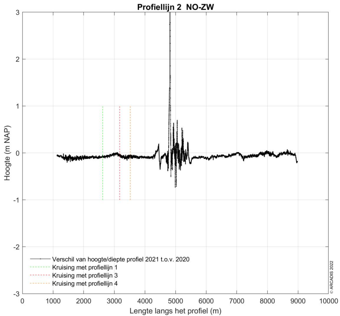
Figuur 4-50 Verschilplot langs profiellijn 2 van noordoost naar zuidwest voor de hoogte/diepte raai meetgegevens van 2020 en 2021. Een positieve waarde betekent dat de hoogte/diepteraai van mei 2021 hoger ligt dan de hoogte/diepteraai van 2020.
