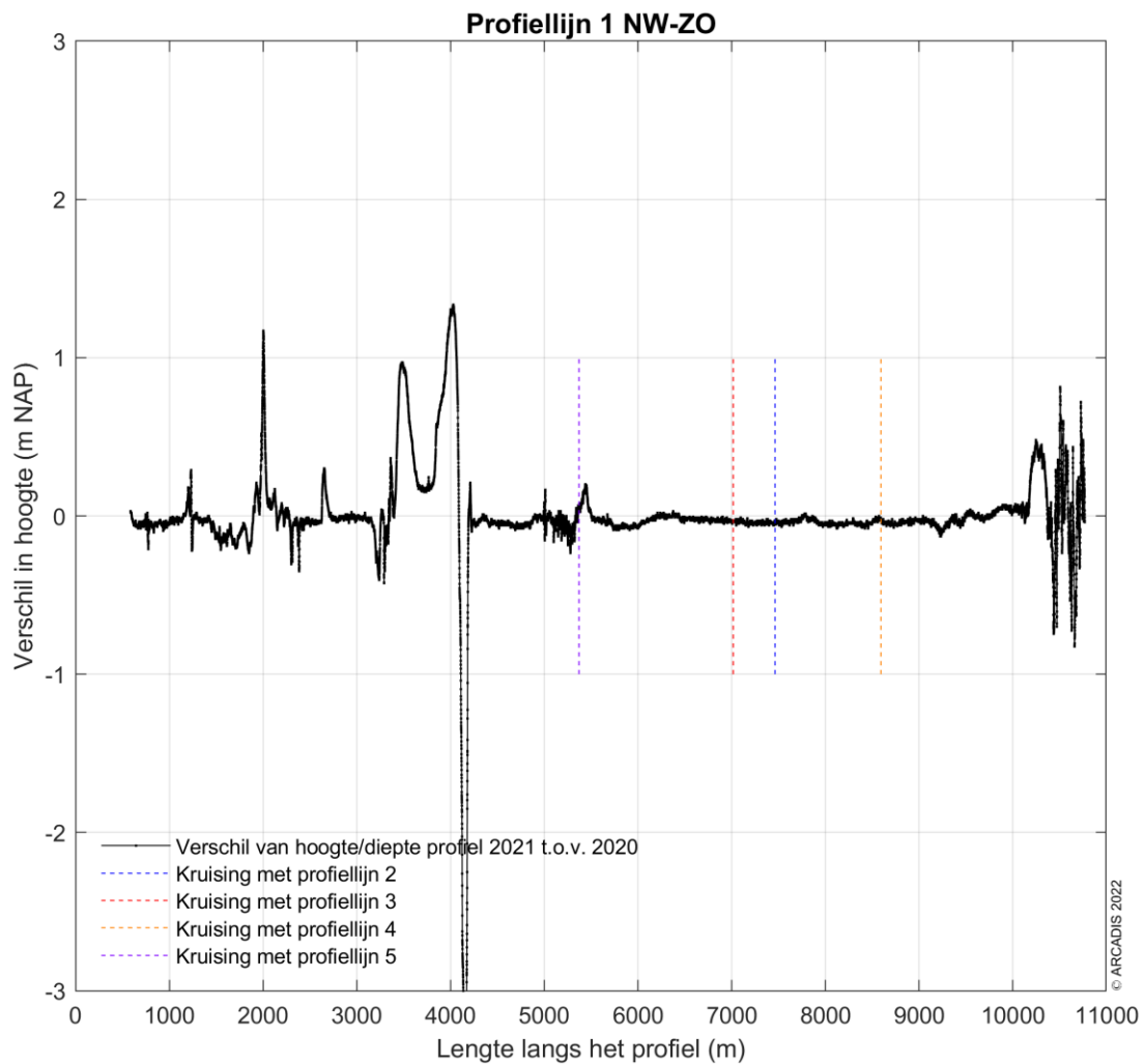
Figuur 4-47 Vershilplot langs profiellijn 1 van noordwest naar zuidoost voor de hoogte/diepte raai meetgegevens van 2020 en 2-21. Een positieve waarde betekent dat de hoogte/diepteraai van 2021 hoger ligt dan de hoogte/diepteraai van 2020.
