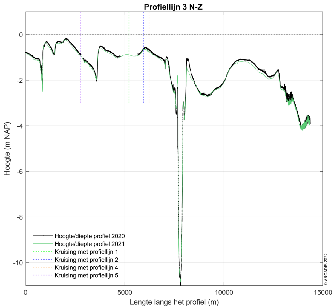
Figuur 4-52 Dwarsprofiel langs profiellijn 3 van noord naar zuid voor de hoogte/diepte raai meetgegevens van 2020 en 2021.
