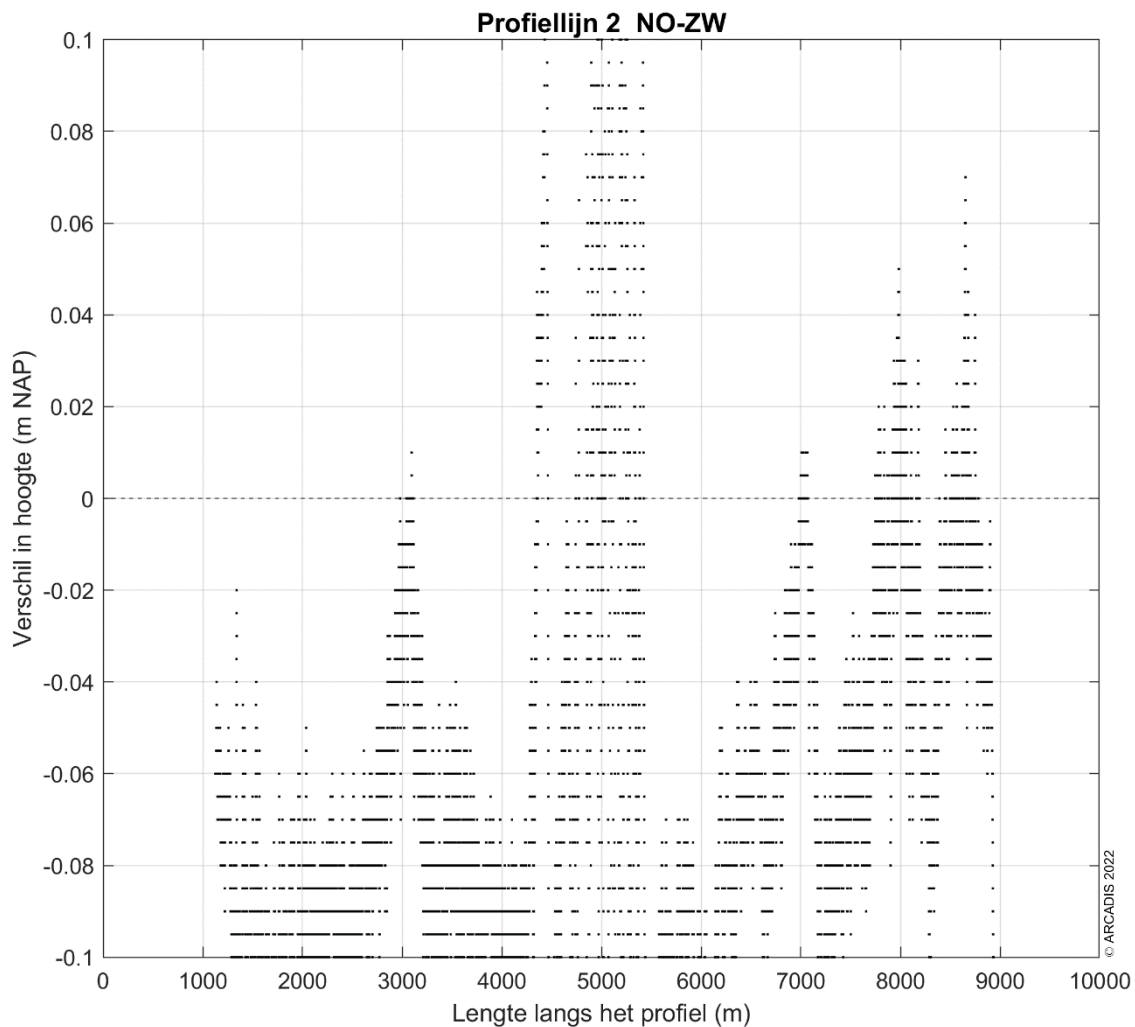
Figuur 4-51 Ingezoomde verschilplot langs profiellijn 2 van noordoost naar zuidwest voor de hoogte/diepte raai meetgegevens van 2020 en 2021. Een positieve waarde betekent dat de hoogte/diepteraai van 2021 hoger ligt dan de hoogte/diepteraai van 2020.
