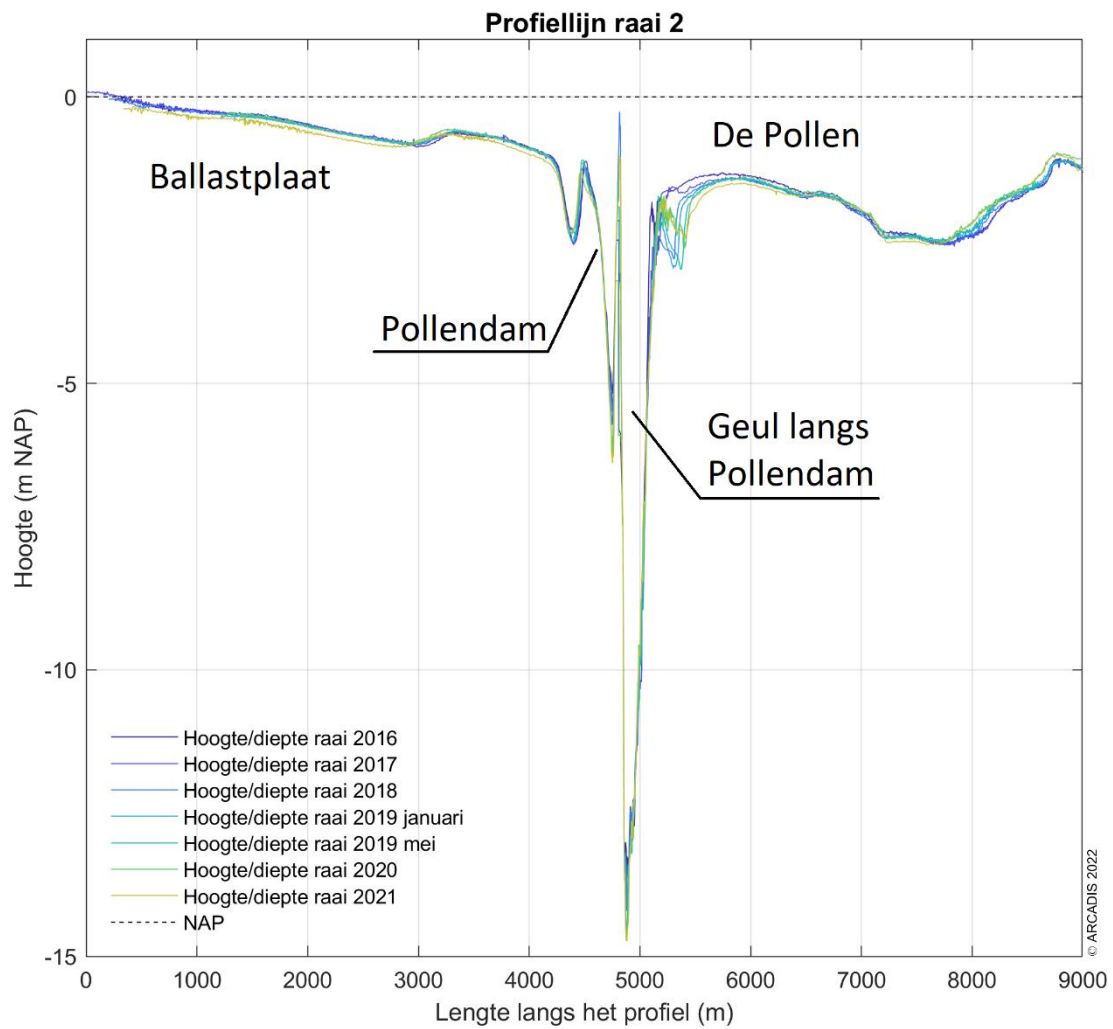
Figuur 5-4 Dwarsprofiel langs profiellijn 2 van noordoost naar zuidwest voor de hoogte/diepte raai meetgegevens van 2016, 2017, 2019, 2020 en 2021.
