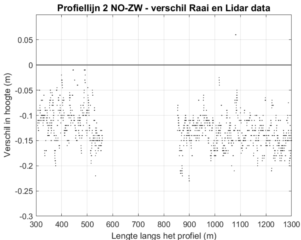
Figuur 0-11 Ingezoomde verschilplot langs profiellijn 2 van noordoost naar zuidwest voor de hoogte/diepte raai meetgegevens van 2016 en de LiDAR-data van 2016. Een positieve waarde betekent dat de LiDAR lager ligt dan de hoogte/diepteraai.
