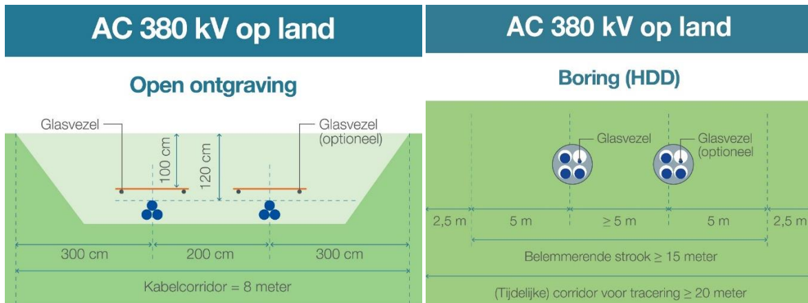
Figuur 3-3 De indicatieve kabelconfiguraties van de open ontgraving en boring voor de 380kV-wisselstroomkabels
