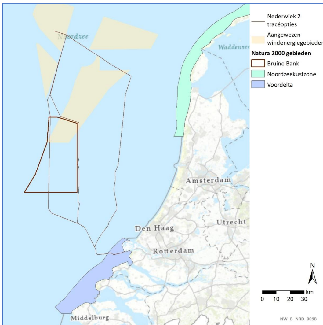
Figuur 3-2 Ligging tracéopties Net op zee Nederwiek 2 ten opzichte van Natura 2000-gebieden
