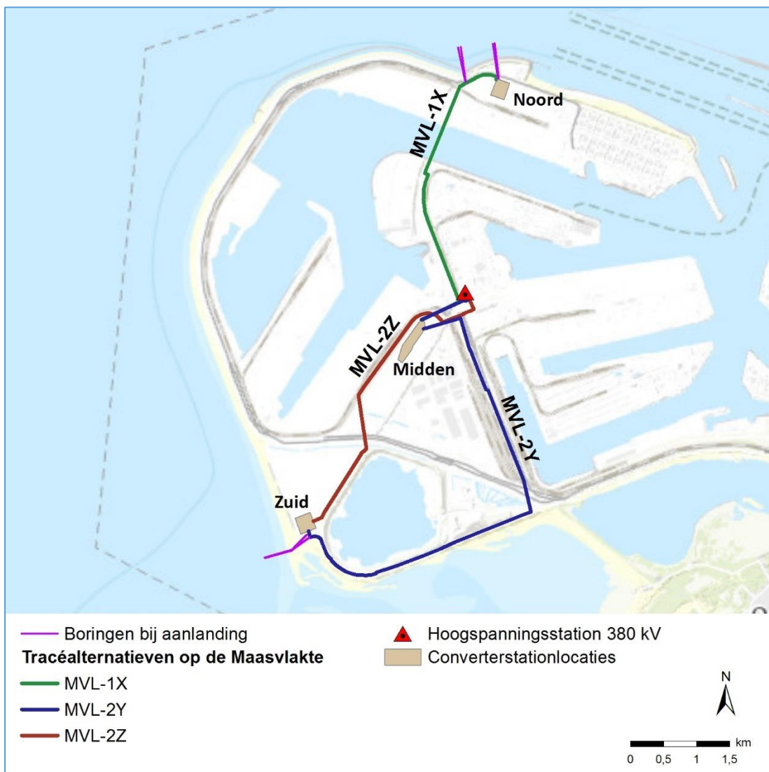
Figuur 2-4 Alternatieven MER fase 1 Net op zee IJmuiden Ver Beta
