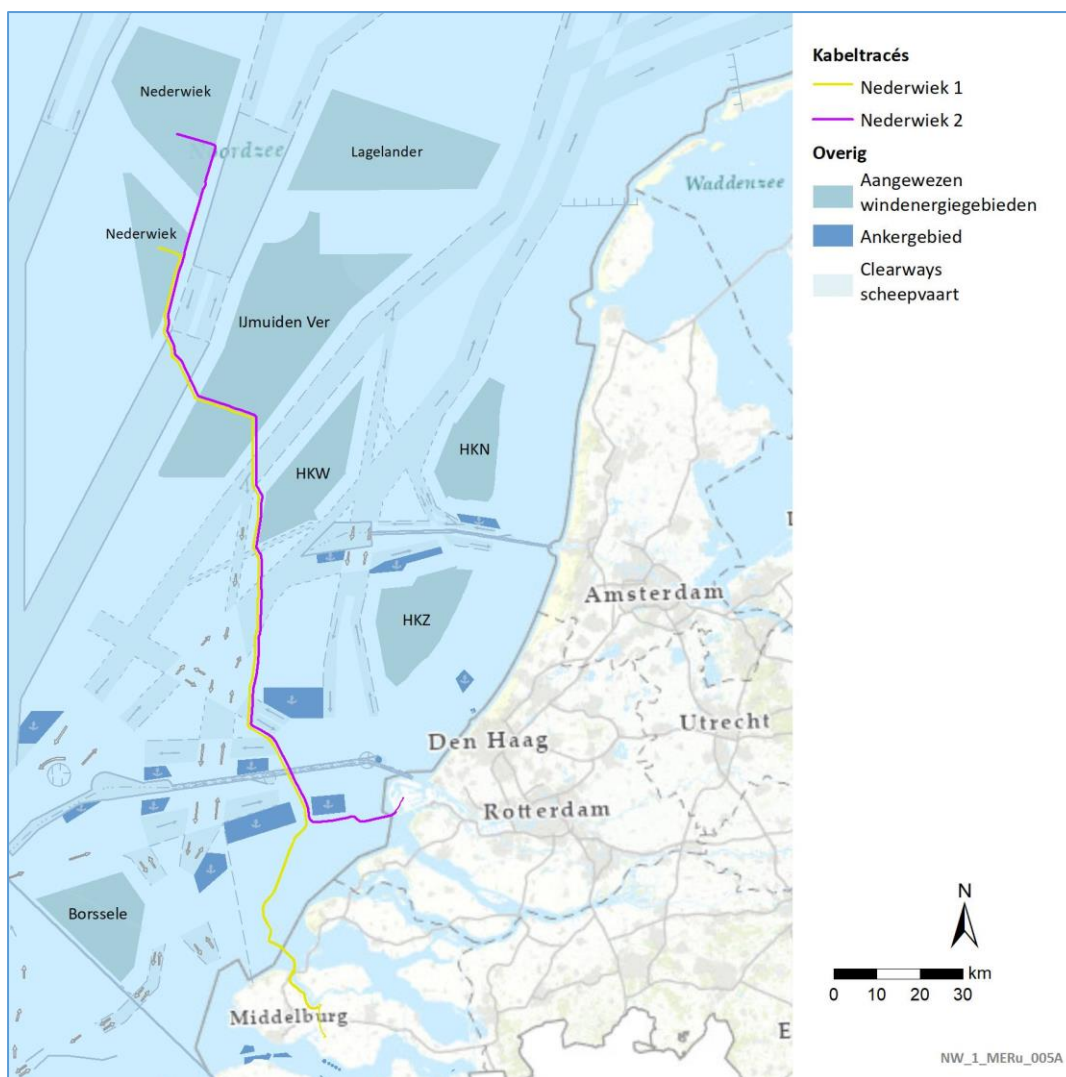
Figuur 1-4 Parallelligging Netten op zee Nederwiek 1 en 2
