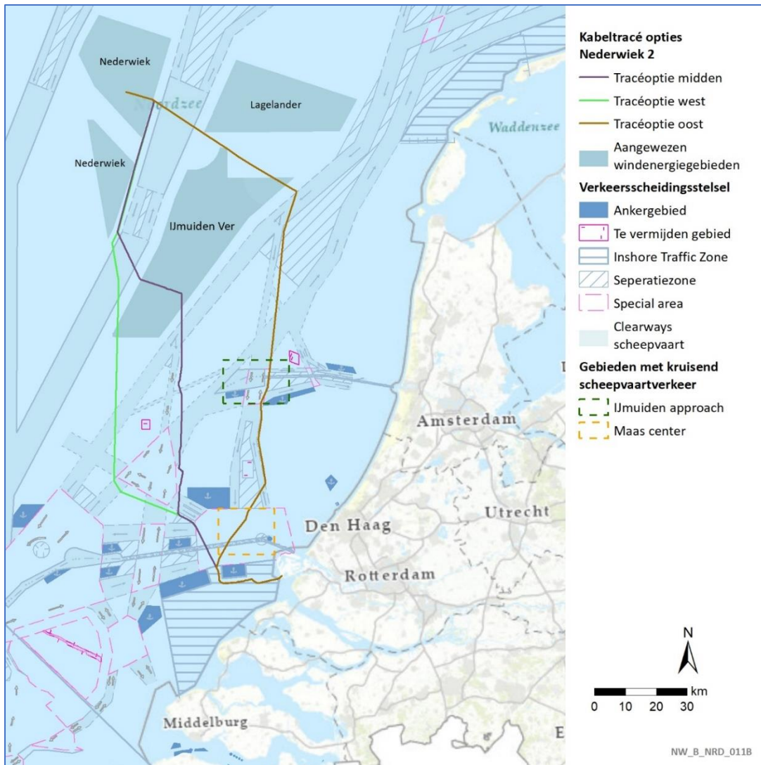
Figuur 3-5 Scheepvaartroutes met Maas Center (geel omkaderd) en het gebied ten noorden van Ijmuiden Approach (groen omkaderd)
