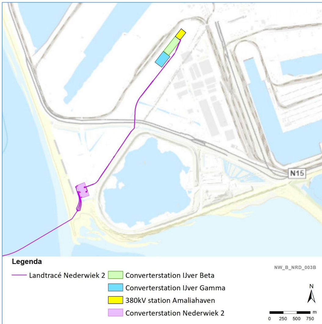
Figuur 2-7 Het landtracé 'midden door' de Maasvlakte
