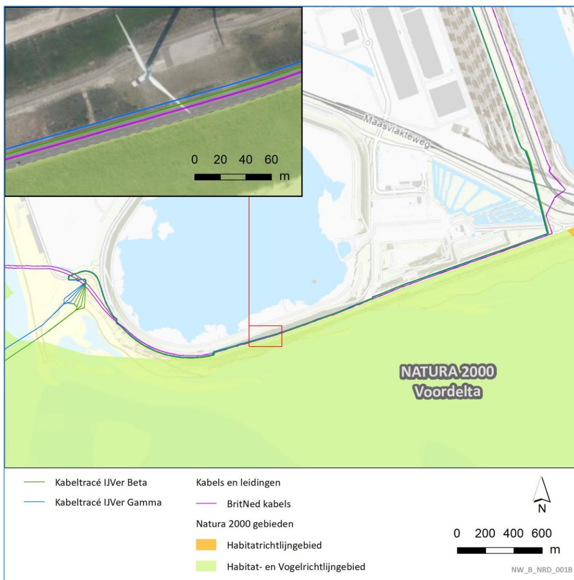
Figuur 2-6 De parallelligging van Netten op zee IJmuiden Ver Beta en Gamma langs Natura 2000-gebied Voordelta
