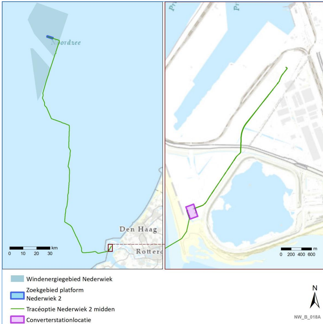
Figuur 4-7 Voorkeurstracé Net op zee Nederwiek 2
