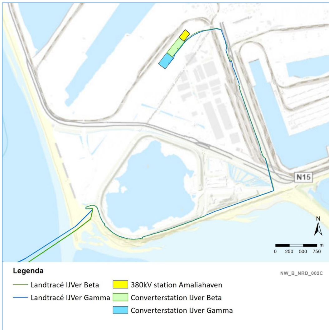
Figuur 2-5 Parallellegging op land Netten op zee IJmuiden Ver Beta en Gamma
