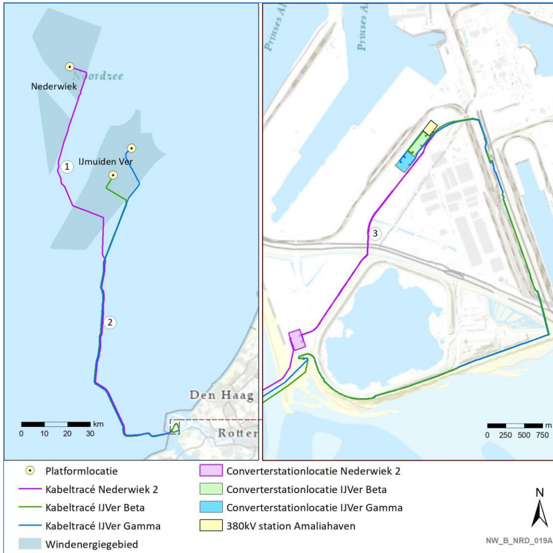
Figuur 1-6 Parallelligging Netten op zee IJmuiden Ver Beta, Gamma en Nederwiek 2
