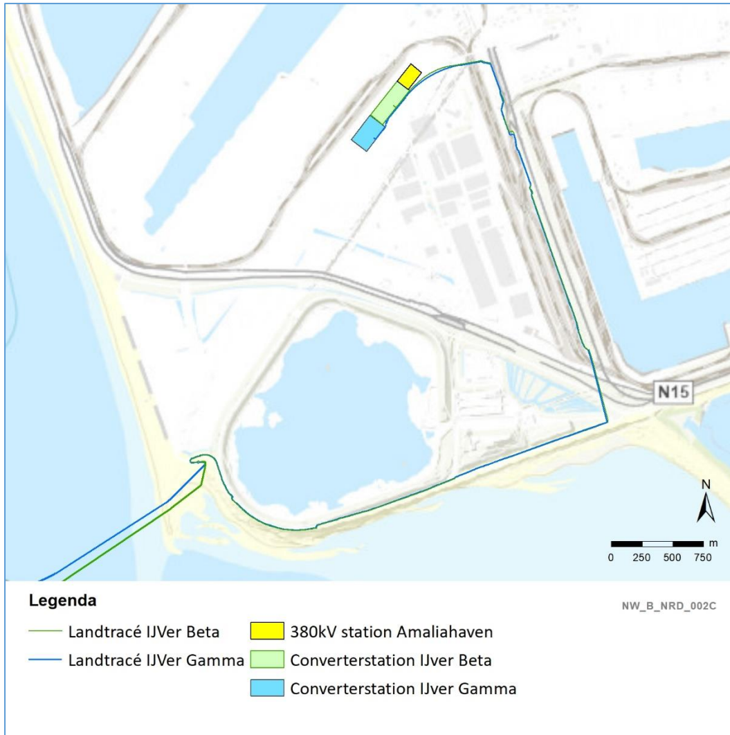
Figuur 4-5 Landtracés Netten op zee IJmuiden Ver Beta en Gamma
