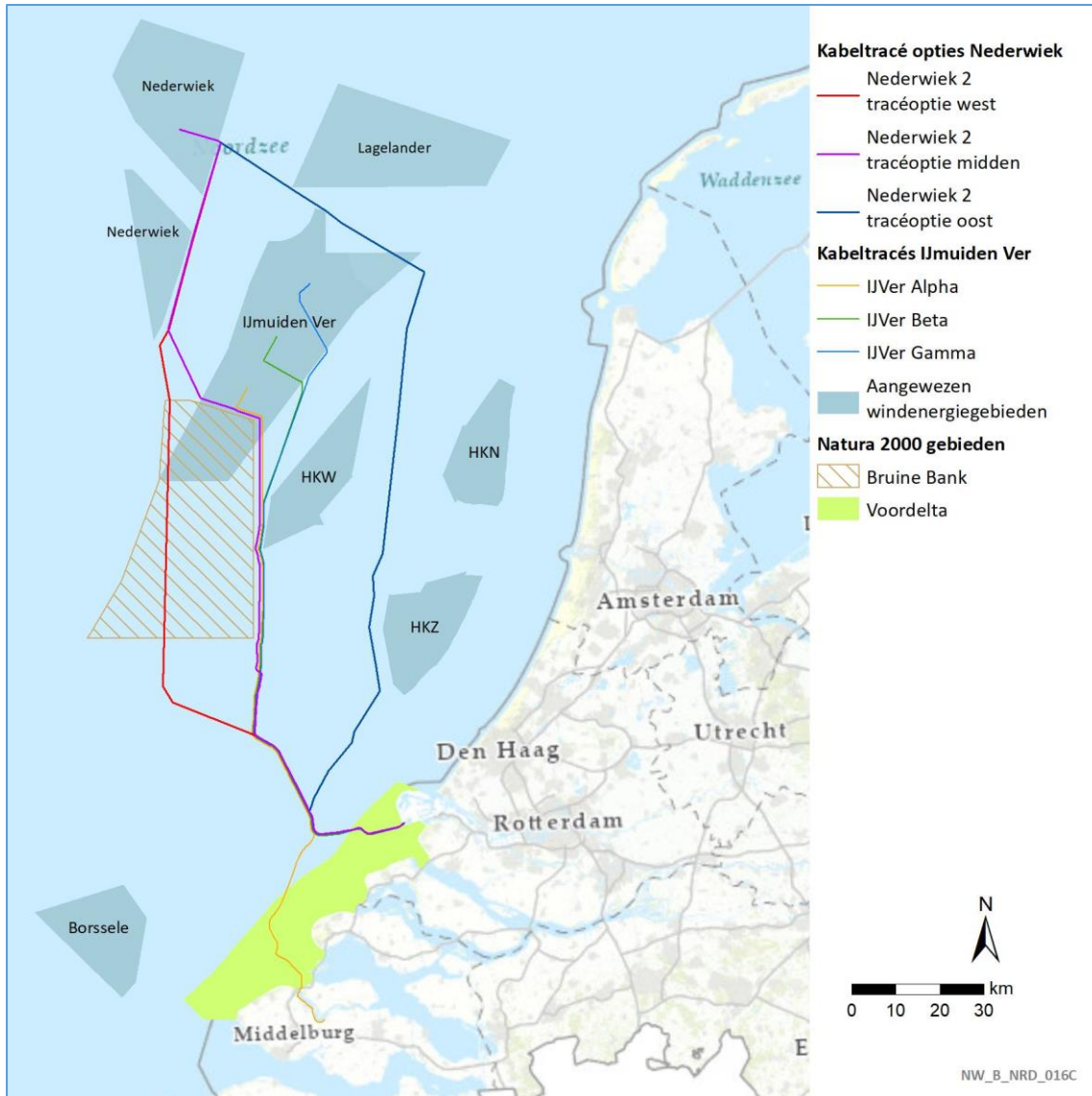
Figuur 2-3 Weergave van het windenergiegebied met de tracéopties op zee van Net op zee Nederwiek 2
