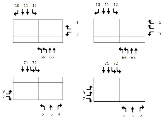
Figuur 4.8 – Vormgeving kruispunt 4 (VRI 140): links huidige situatie; rechts autonome situatie die nodig is op basis van eerdere berekeningen
