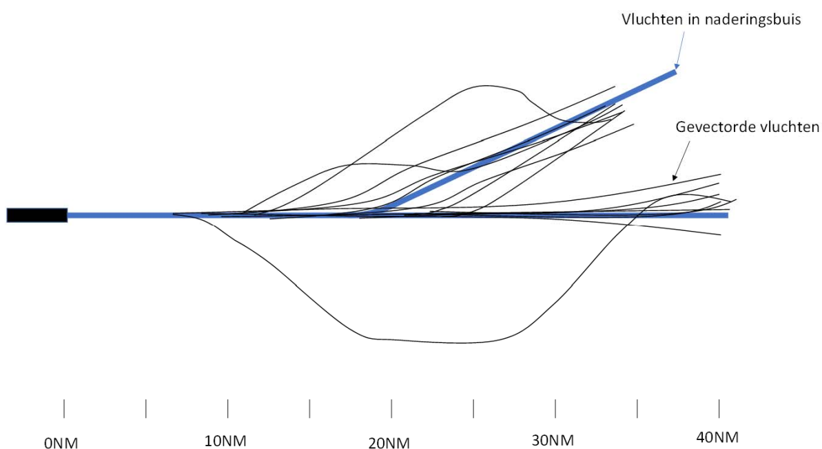
Figuur 3-5 Bovenanzicht van gevectorde vluchten en vluchten in naderingsbuis
