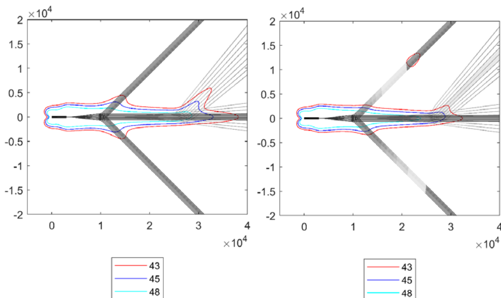
Figuur 12-5 De 43 dB(A), 45 dB(A) en 48 dB(A) contouren en de gevlogen vliegpaden van 50.000 vertrekkende en 50.000 naderende op de generieke start- en landingsbaan in één jaar overdag. Links geeft de resultaten voor de referentiesituatie en rechts geeft de resultaten voor het alternatief Vast
