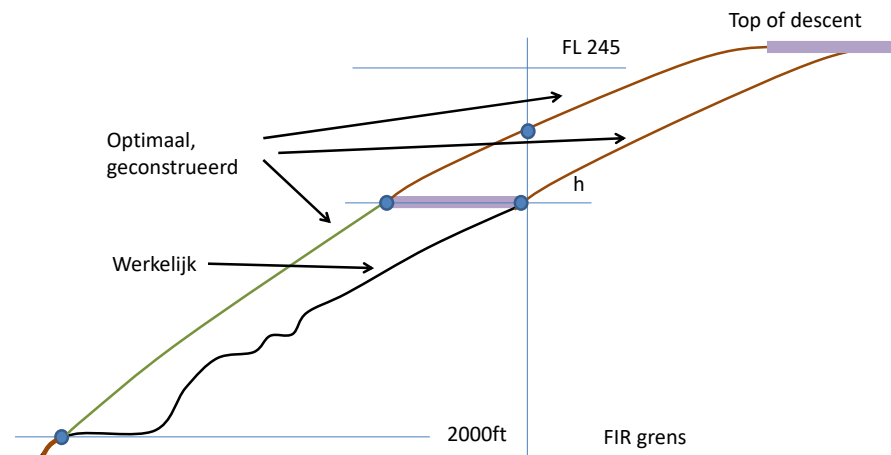
Figuur 11-3 - Beschouwd wordt een vlucht die over het kortste horizontale pad vliegt. Het hoogteprofiel van het relevante deel van de vlucht (tussen 2000voet en FL245 en binnen het Nederlands luchtruim) is in zwart aangegeven ("werkelijk").
