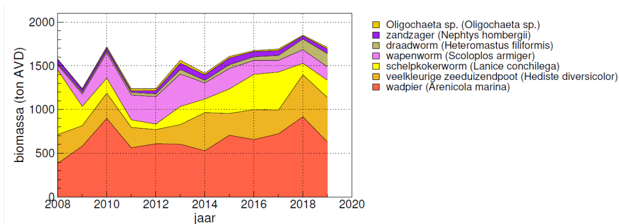
Figuur 9-7. Ontwikkeling van de totale biomassa wormen (in tonnen asvrij drooggewicht) in de kombergingen van Pinkegat-Zoutkamperlaag in de zomer, onderverdeeld naar de verschillende wormensoorten.
