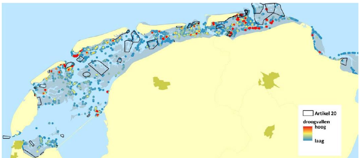
Figuur 10-2. Puntdichtheidskaart van droogvallers tijdens het vaarseizoen 2017 voor het gehele Waddengebied op basis van AIS. Ook aangegeven de grenzen van artikel 20 gebieden, waar droogvallen niet is toegestaan. Bron: (Meijles et al. 2018b).
