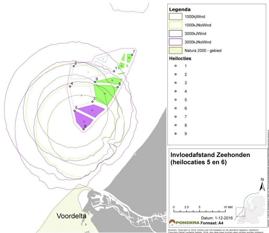
Figuur 6.4 Overlap van verstoringscontouren van zeehonden met de Natura 2000-gebieden Voordelta en Vlakte van de Raan door heien, zonder toepassen van een geluidsnorm, voor de aanleg van kavel III van windpark Hollandse Kust (zuid).
