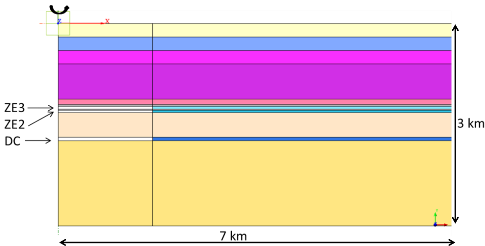
Figuur 5: De geometrie van het gebruikte eindig-elementen model. De locatie van de carbonaaten- en zandsteen reservoirs is aangegeven.
