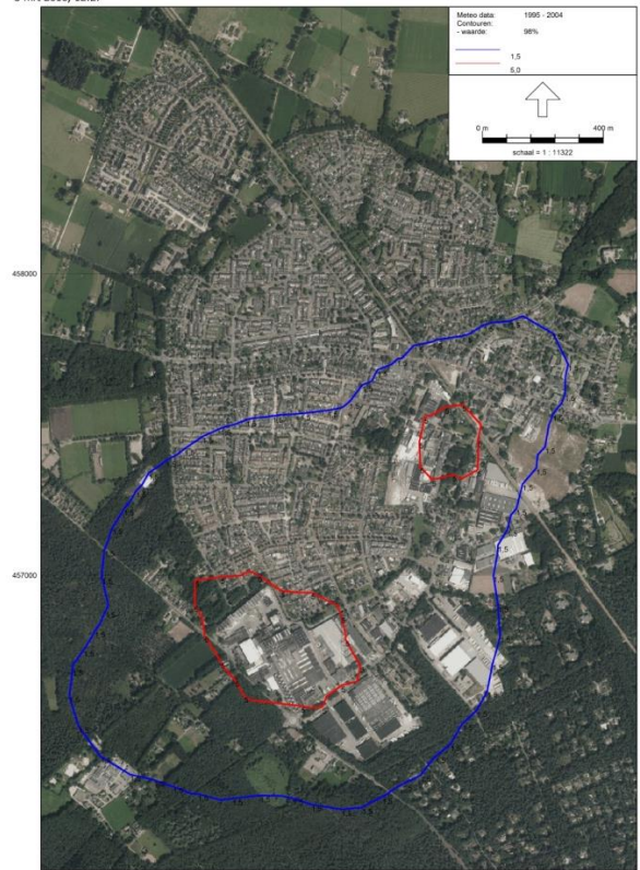
Figuur b: Contouren van 5 en 1,5 ou E /m 3 als 98-percentielwaarde in de vergunde situatie met maximale inzet van nageschakelde technieken 21 (scenario 1).
