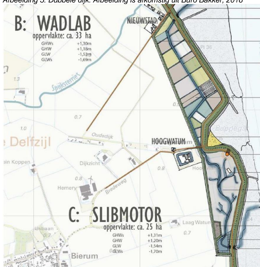
Afbeelding 5: Dubbele dijk. Afbeelding is afkomstig uit Buro Bakker, 2016
