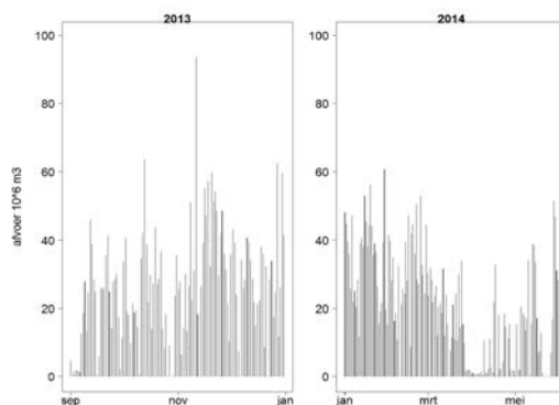
Figuur 3-2 Dagelijkse zoetwater afvoer per dag in 10^6 \text{ m}^3 .
